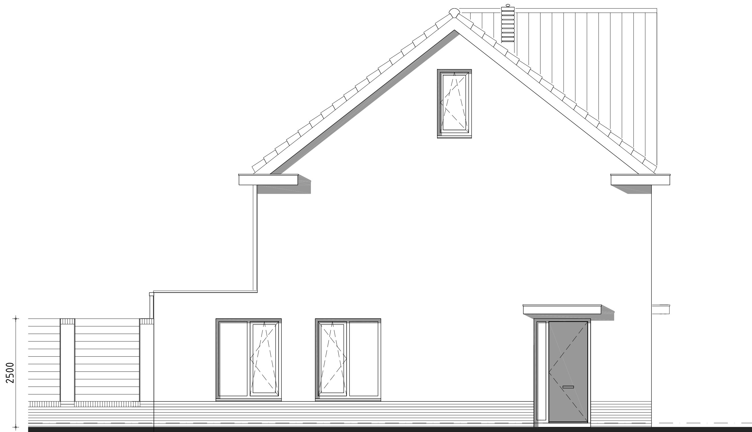
linker zijgevel
