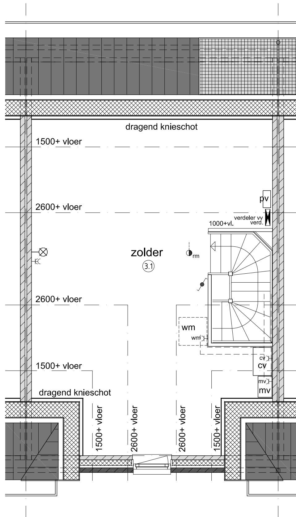
2e verdieping
