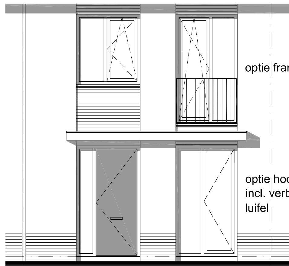
voorgevel
