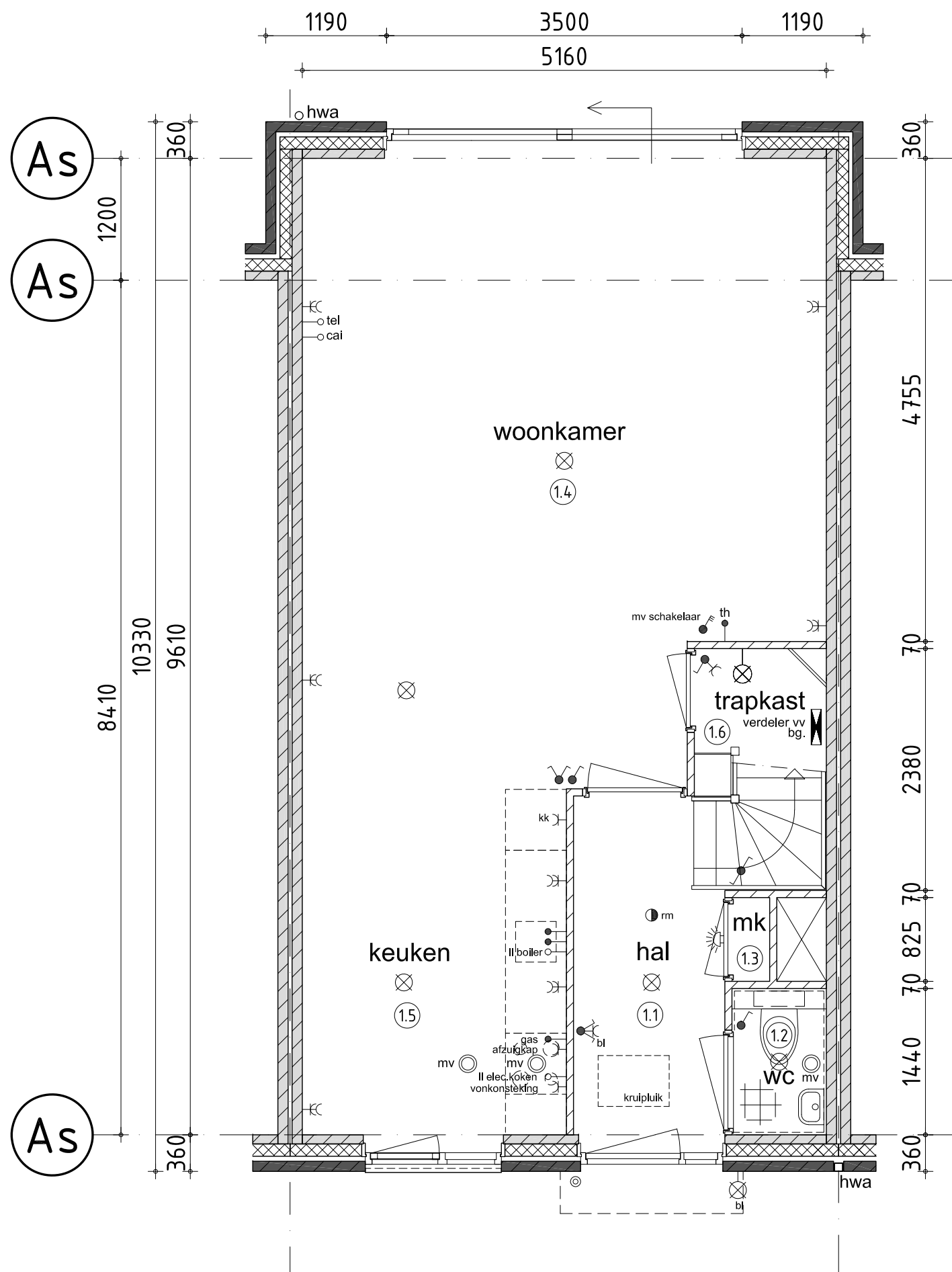
begane grond
