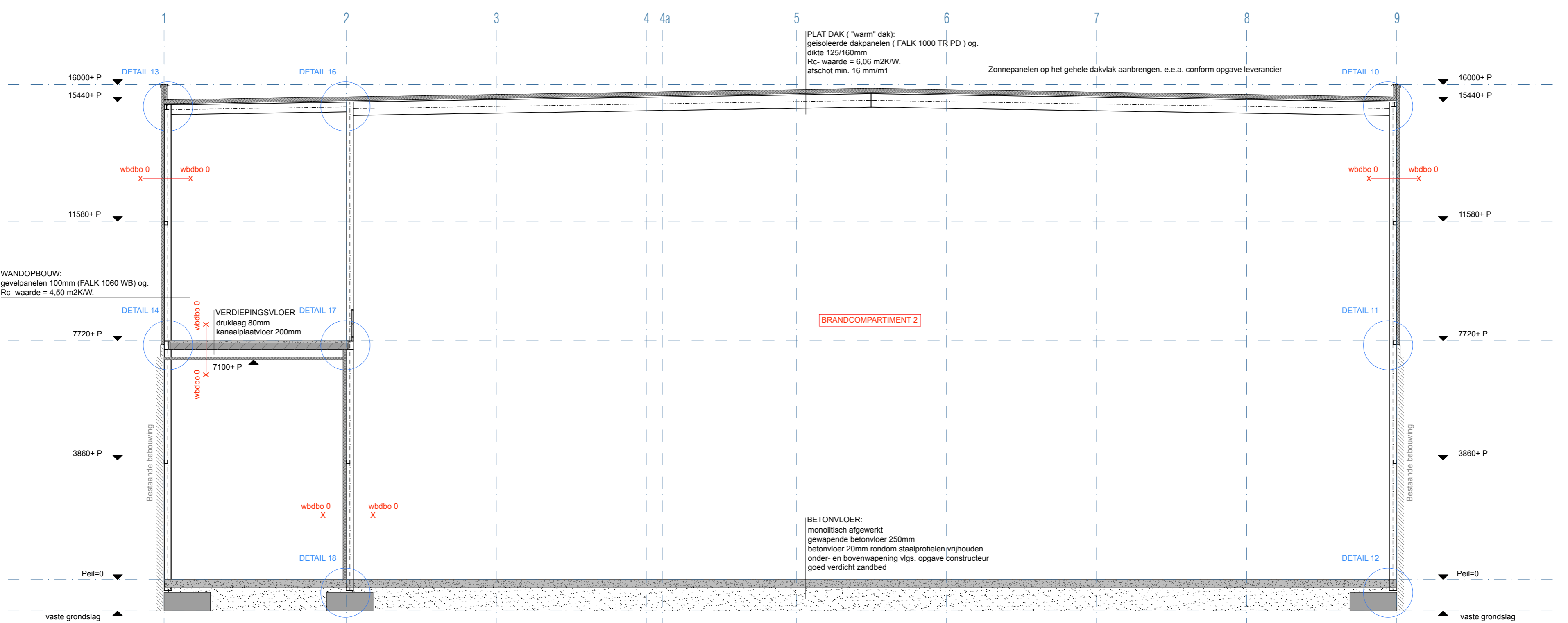
DOORSNEDE BB
