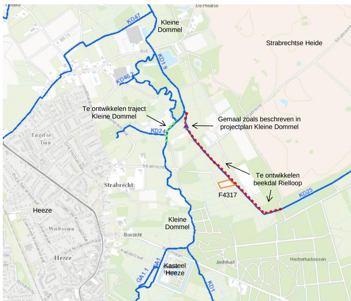
Figuur 1, overzichtstekening
