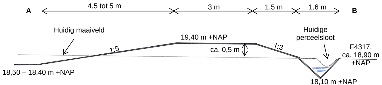
Figuur 18, dwarsprofiel maatregelen rondom perceel F4317, hoogten zijn t.o.v. NAP
