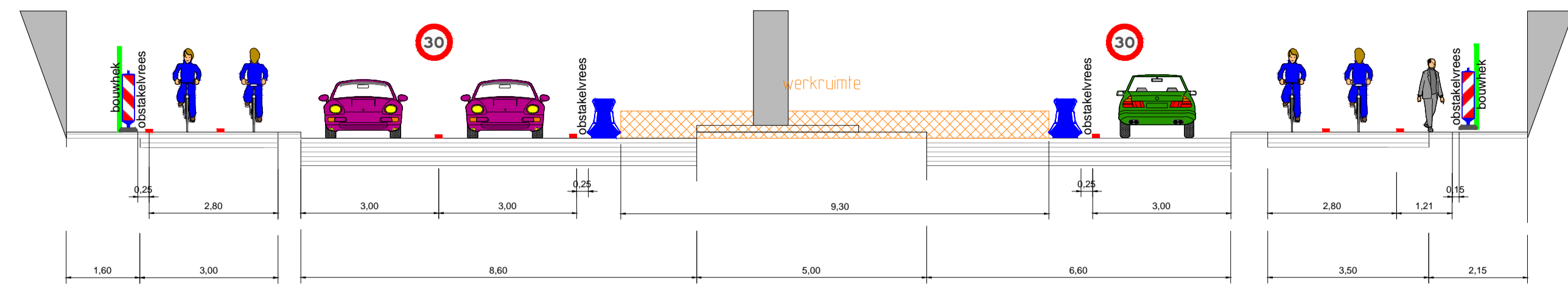
Dwarsdoorsnede A - a
