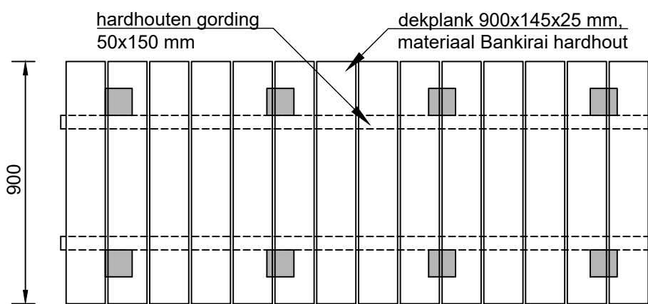
BOVENAANZICHT VLONDERBRUG
