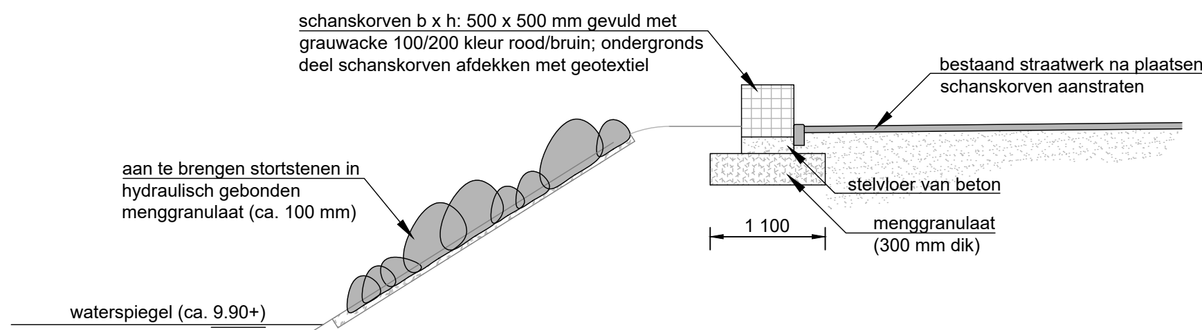
Detail 1 principe schanskorven bij brug Raadhuisstraat schaal 1:50
