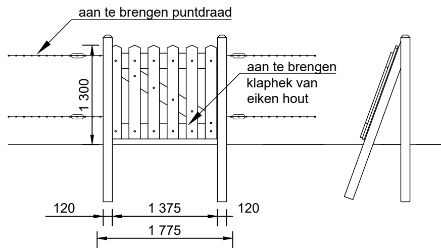
Detail klaphek schaal 1:50
