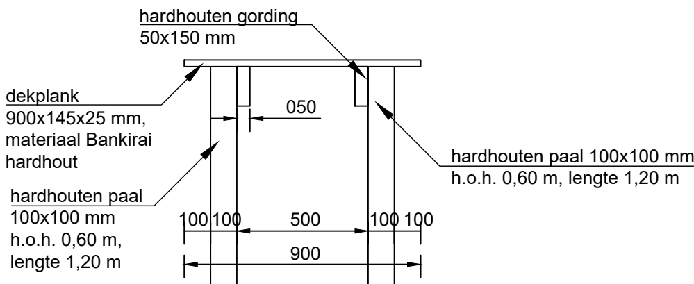
DWARSDOORSNEDE VLONDERBRUG
