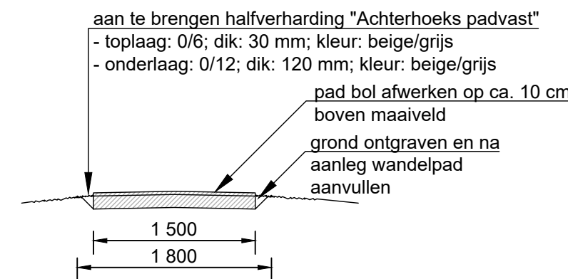
Detail padvast halfverharding bij ontgraving schaal 1:50
