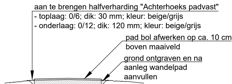
Detail padvast halfverharding bij ontgraving schaal 1:50
