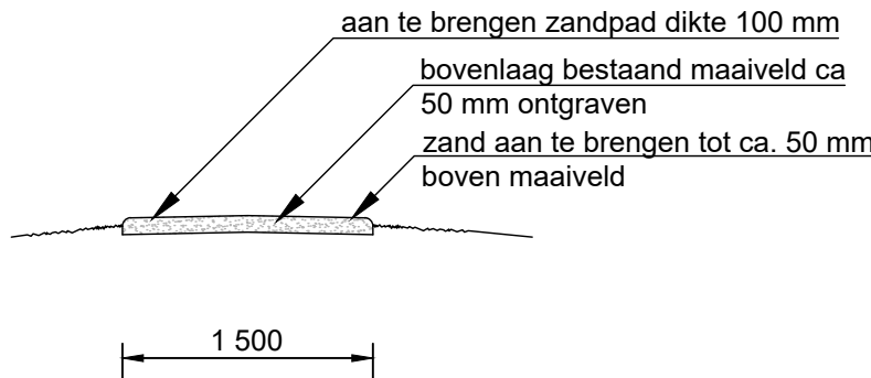
Detail zandpad schaal 1:50
