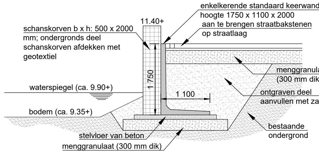
Detail 2 principe schanskorven centrum park schaal 1:50
