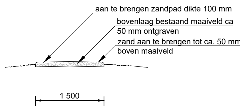
Detail zandpad schaal 1:50
