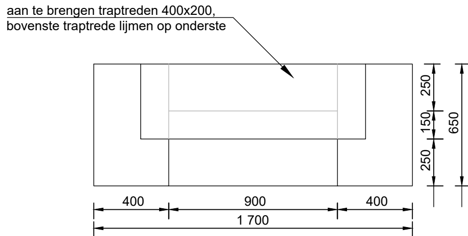
Detail traptreden schaal 1:20
