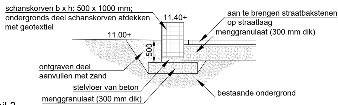
Detail 3 principe schanskorven centrum park schaal 1:50
