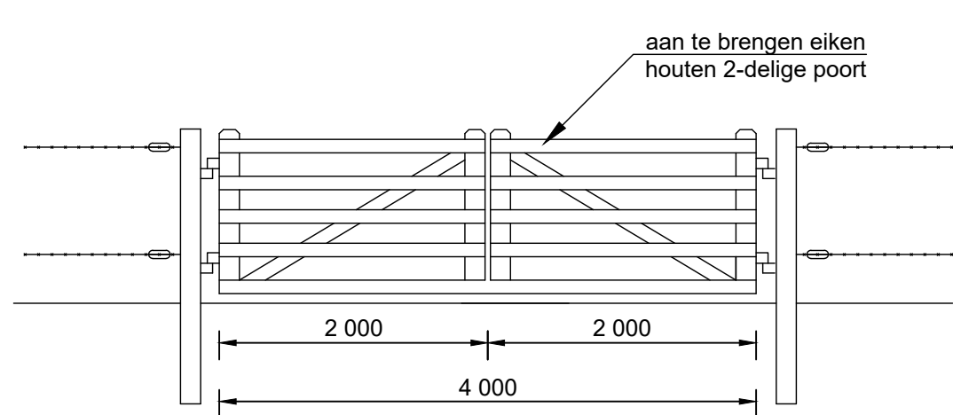
Detail 2-delige poort schaal 1:50
