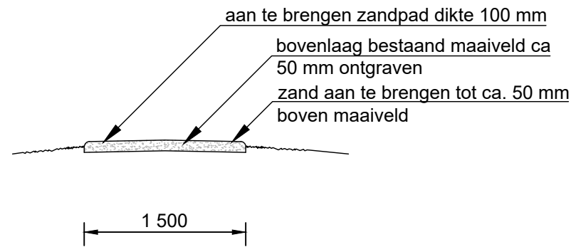
Detail zandpad schaal 1:50
