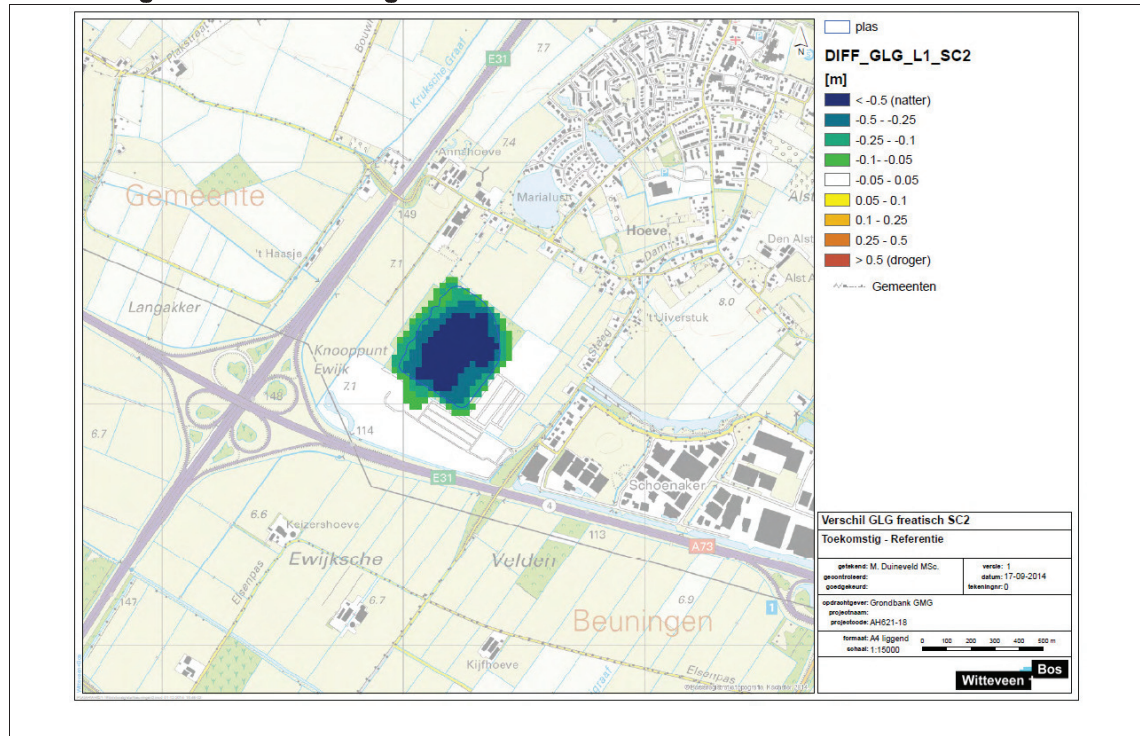
Afbeelding 3.21. Verandering GLG
