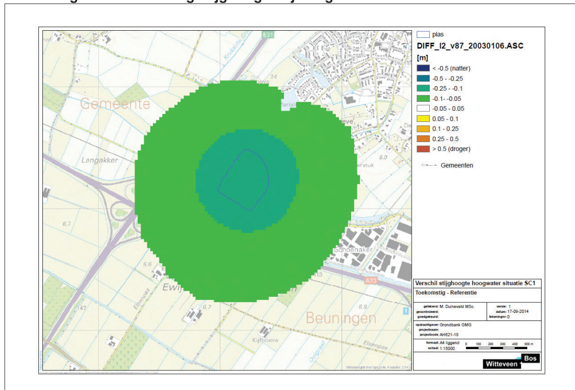
Afbeelding 3.9. Verandering stijghoogte bij hoogwater
