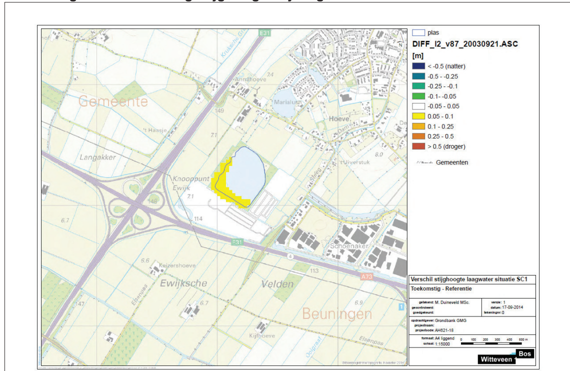
Afbeelding 3.8. Verandering stijghoogte bij laagwater
