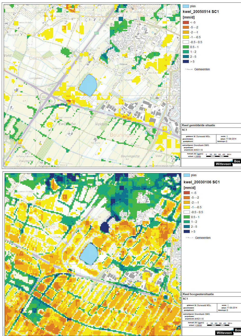
Afbeelding I.3. Kwel scenario 1
