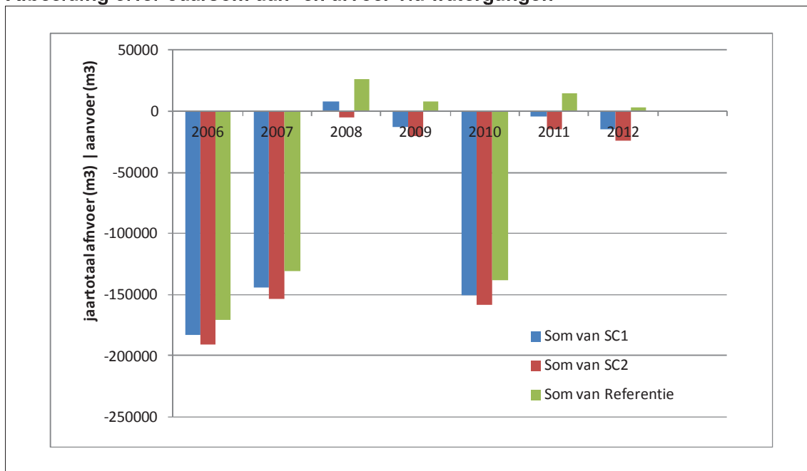
Afbeelding 3.18. Jaarsom aan- en afvoer via watergangen
