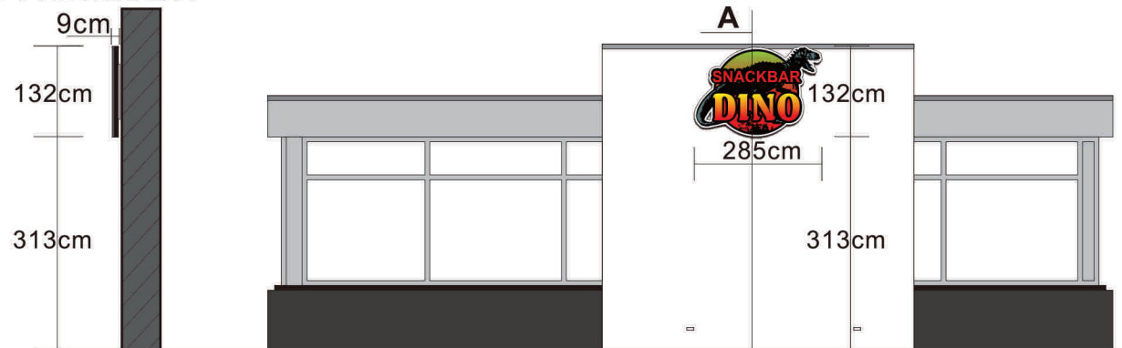
RECHTERZIJGEVEL
