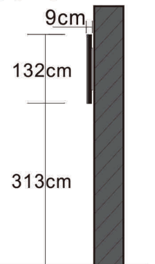
DOORSNEDE B
