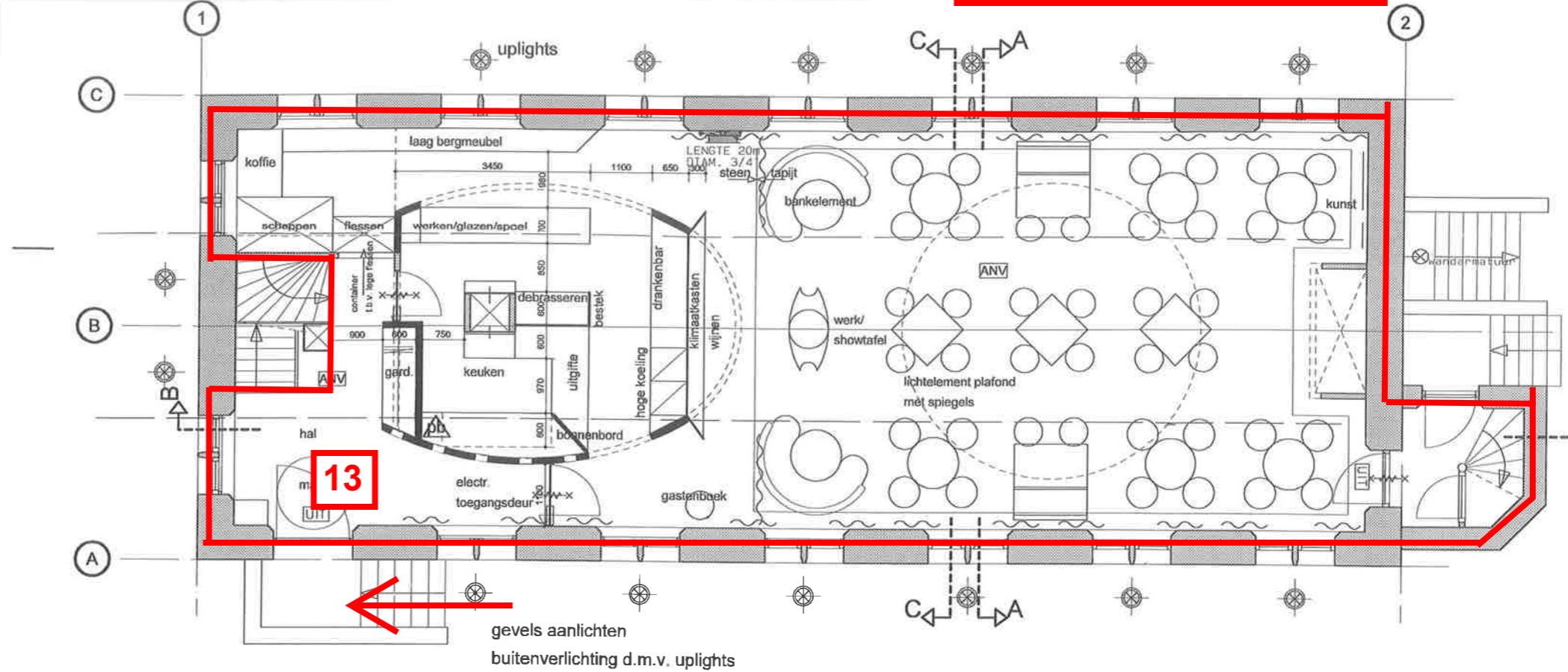
begane grond
