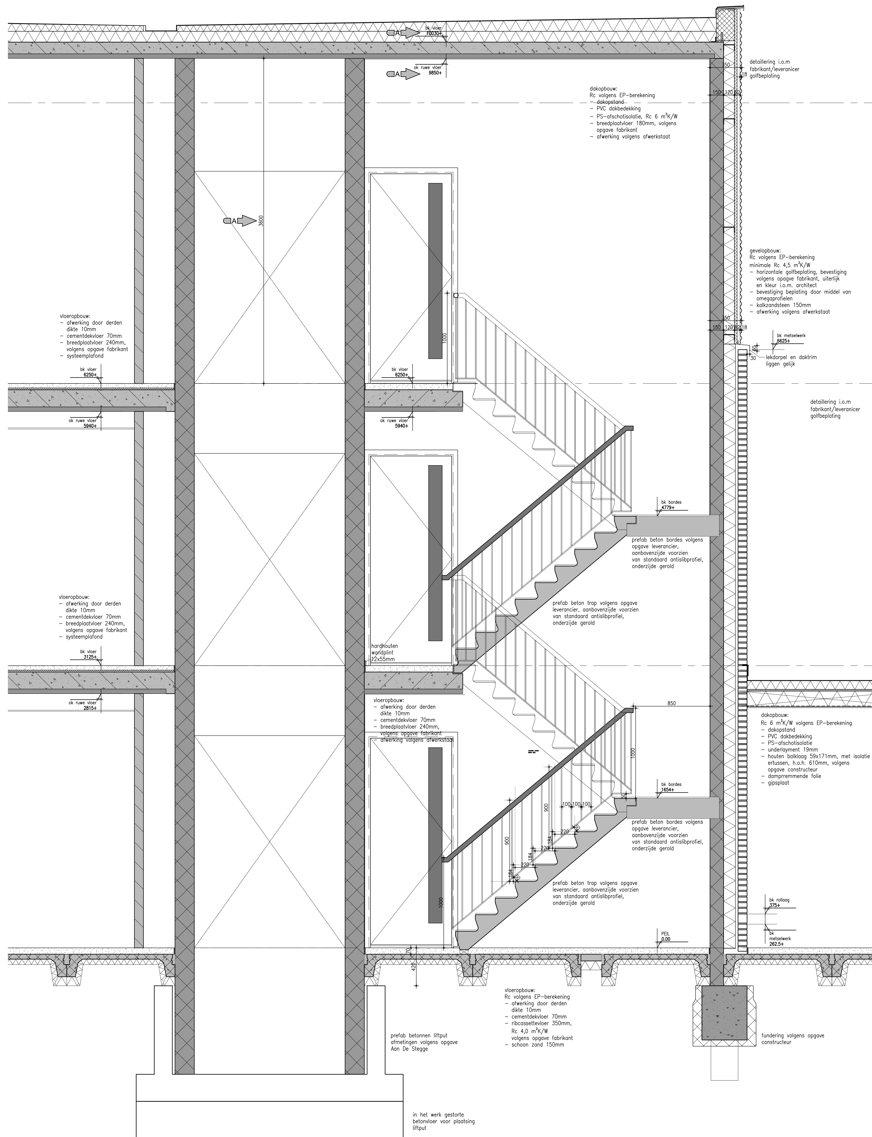
DOORSNEDE A
