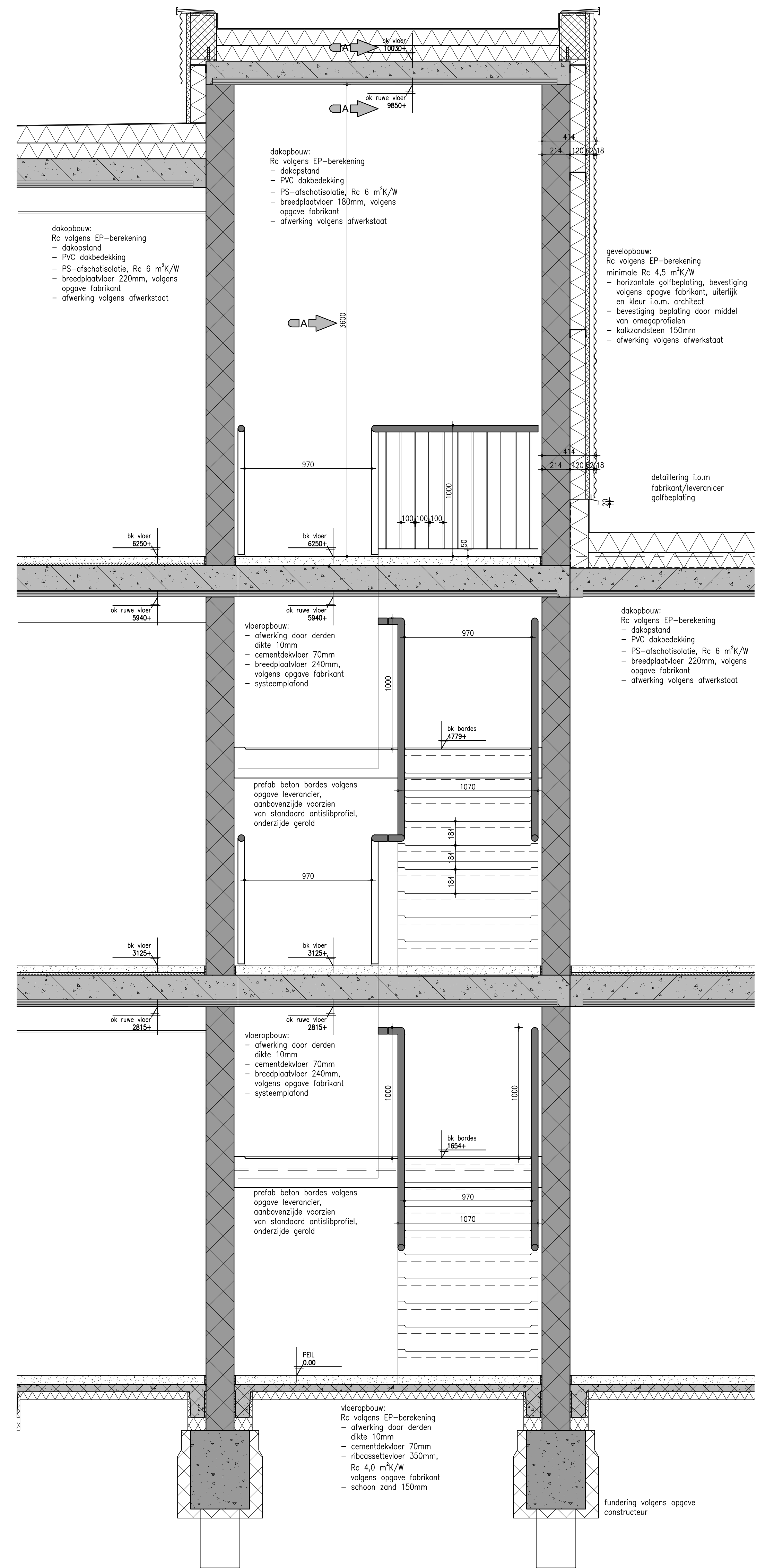
DOORSNEDE B
