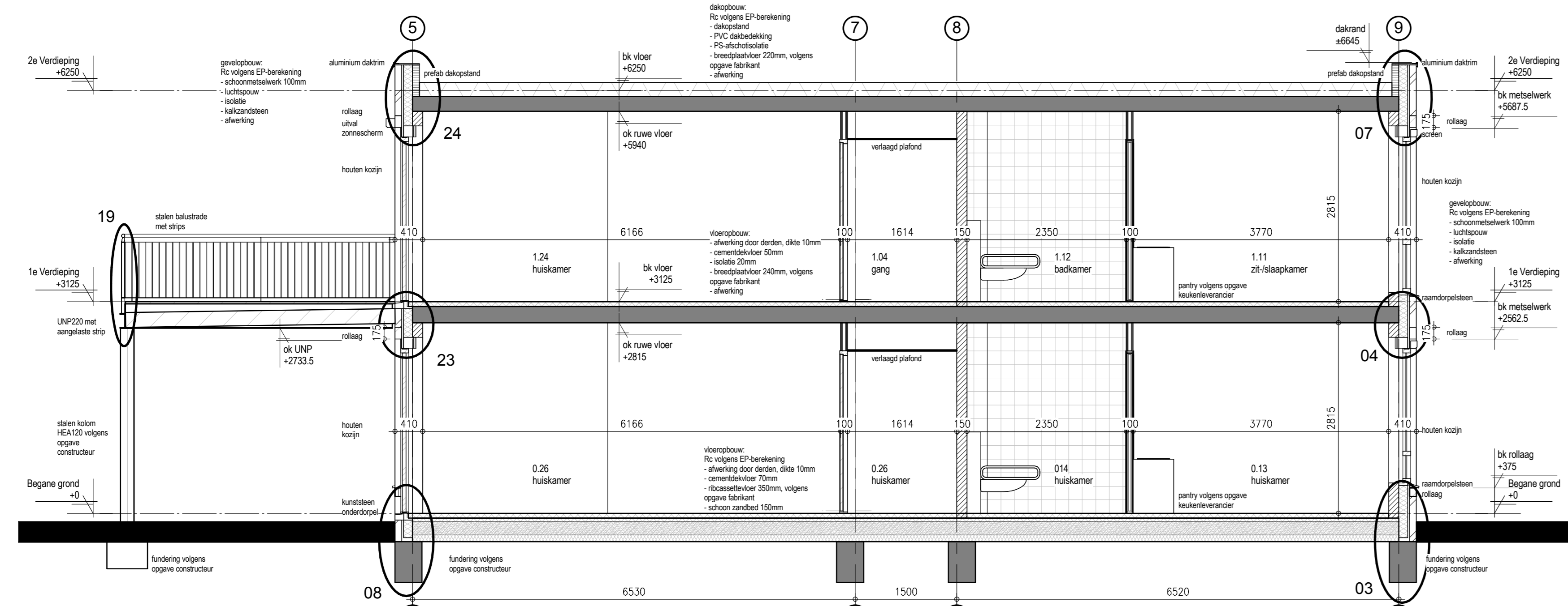
DOORSNEDE C-C
