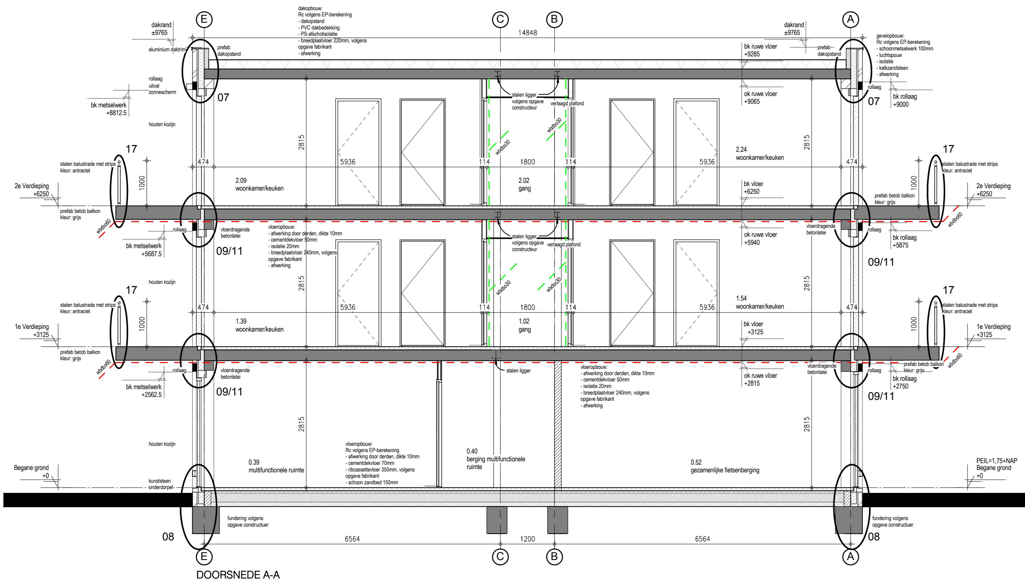
DOORSNEDE A-A
