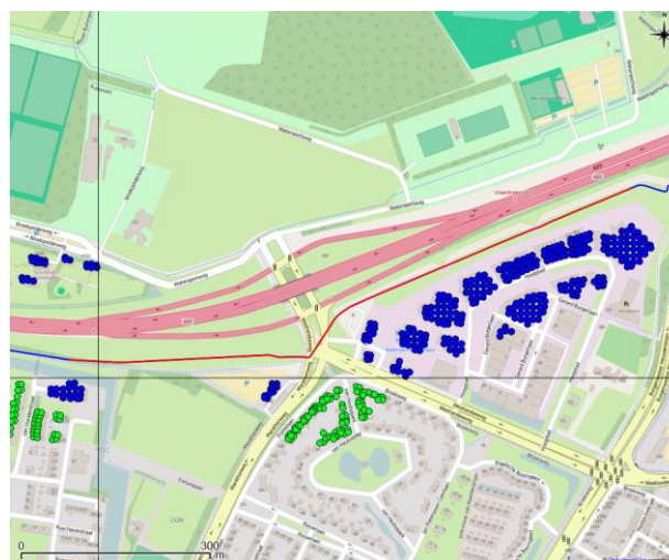
Figuur 10 Ligging kilometer hoogste GR
