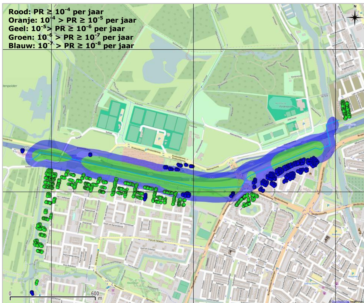
Figuur 3 PR van gastransportleiding W-521-28 (lichtblauw) in de huidige situatie.
