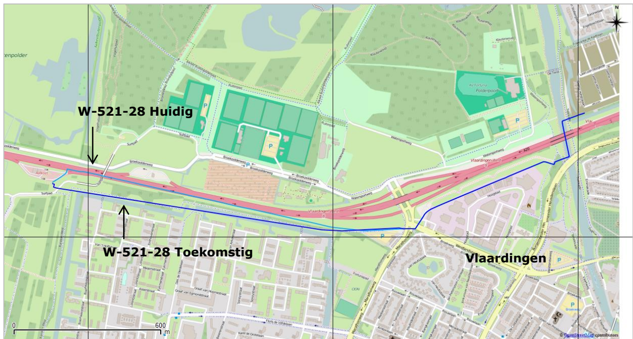
Figuur 1 Ligging van gastransportleiding W-521-28 vóór (lichtblauw) en ná (donkerblauw) verlegging..
