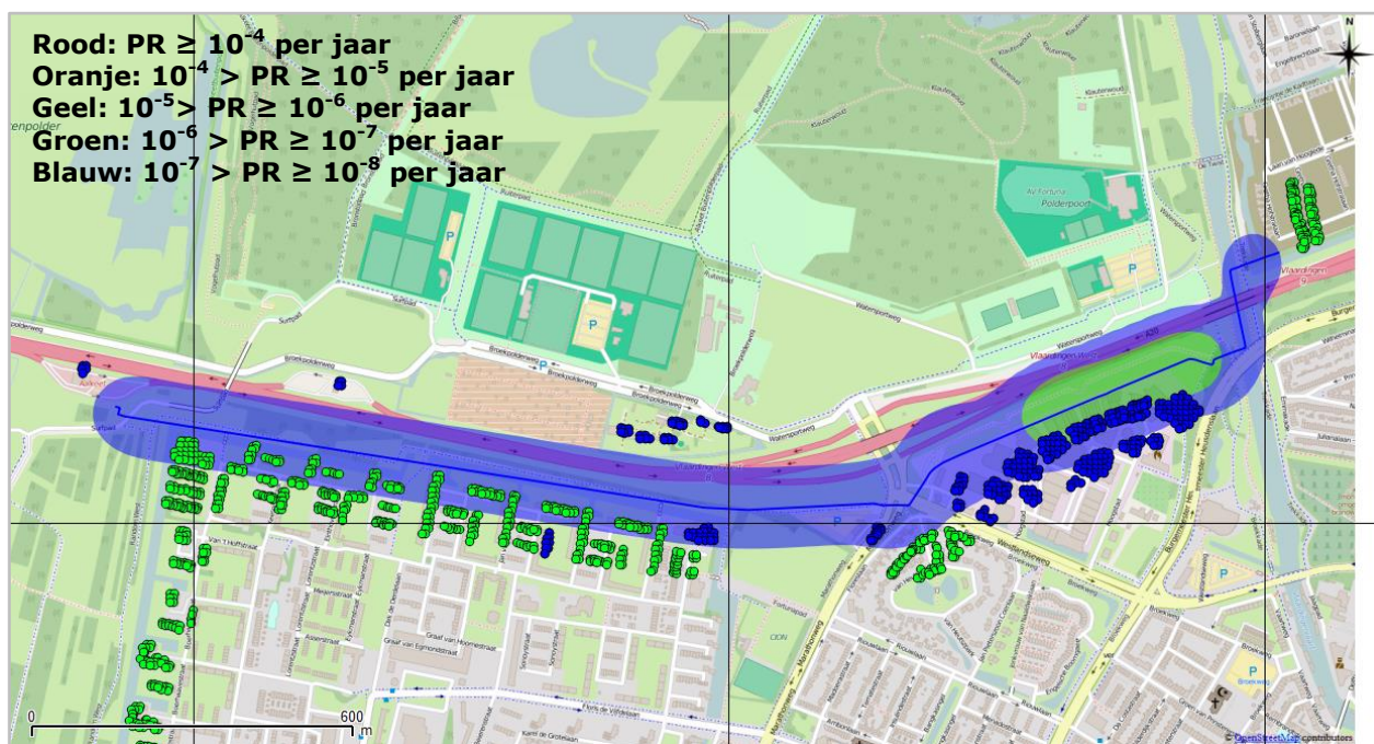
Figuur 4 PR van gastransportleiding W-521-28 (donkerblauw) in de toekomstige situatie.
