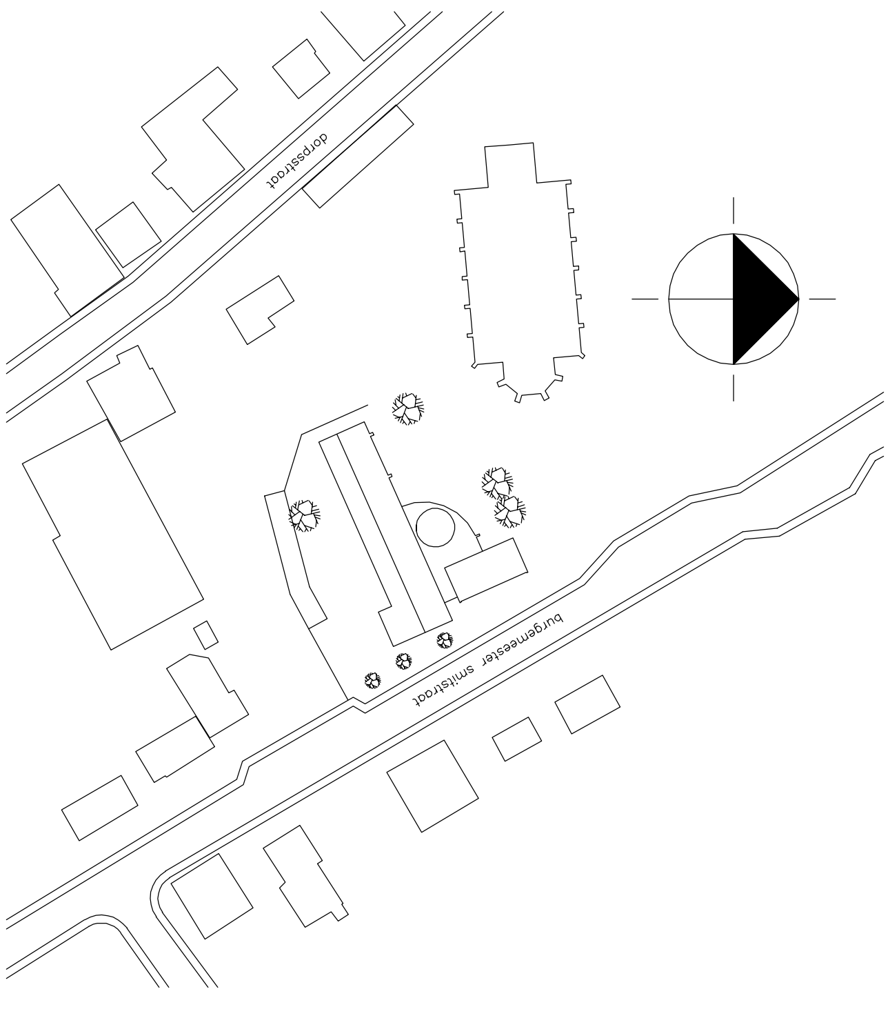
situatie (schaal 1:1000)
