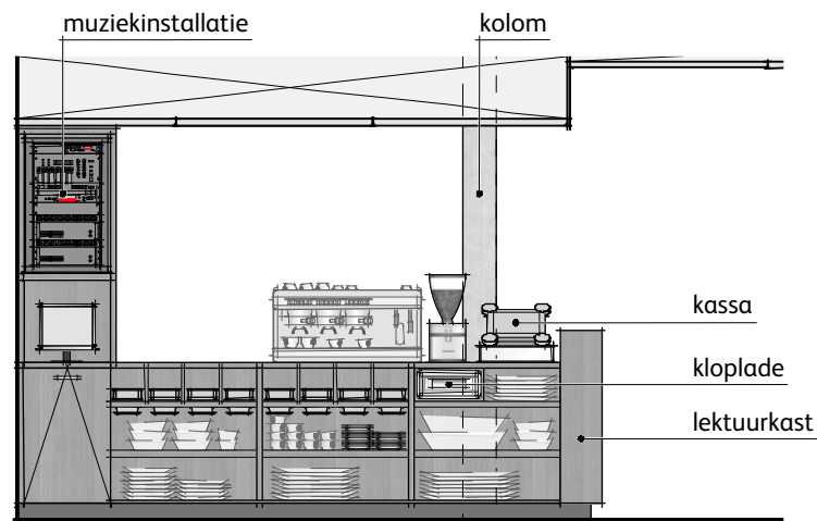
Aanzicht koffiekast 1:50
