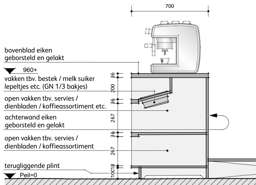
Principe koffiekast 1:20
