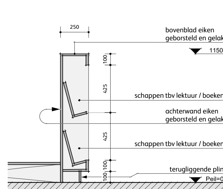
Principe lektuurkast 1:20
