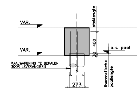
Algemeen paalkopdetail 1:20 (principe)
