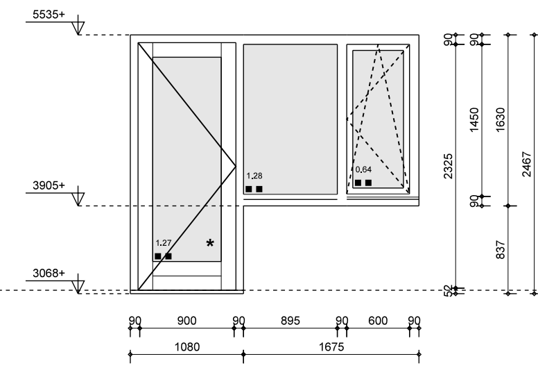
merk D1H als geteind: 1x geproefde: 1x materiaal: hout 90x14mm vulling: geventileerde beglazing, veiligheidsbeglazing (*) deur: Hübner Phoenix laag reflecterend opmerking: intraswerendklasse 2 (NEN 5086)
