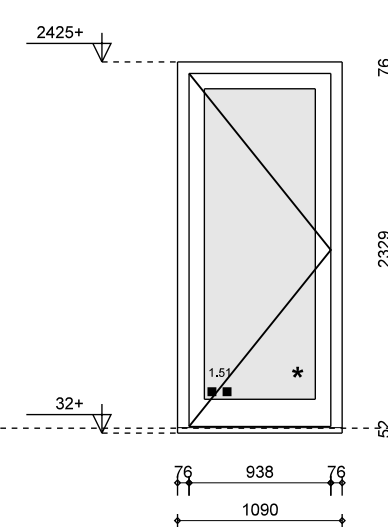
merk D1A als geteind: 1x geproefde: -- materiaal: aluminium deur: aluminium deur x, x, geventileerde veiligheidsbeglazing (*) vulling: geventileerde beglazing opmerking: intraswerendklasse 2 (NEN 5086)
