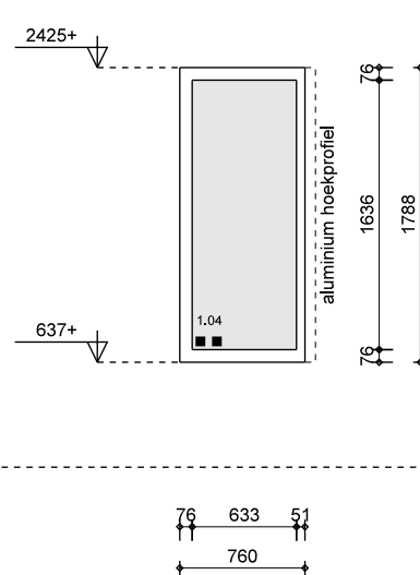
merk A3A als geteind: 1x (x 30 min VDBCO) geproefde: 1x materiaal: aluminium vulling: geventileerde beglazing (1x 30 min VDBCO) opmerking: koppeling met aluminium hoekprofiel
