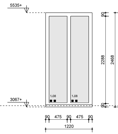
merk I1H als geteind: 1x geproefde: -- materiaal: hout 90x14mm vulling: geventileerde beglazing opmerking: intraswerendklasse 2 (NEN 5086)
