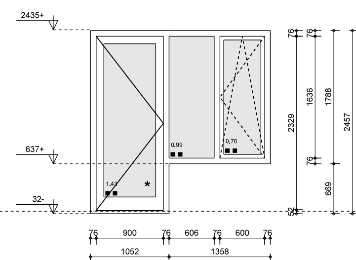
merk F1A als geteind: 2x geproefde: 2x materiaal: aluminium vulling: geventileerde beglazing deur: aluminium deur x, x, geventileerde veiligheidsbeglazing (*) deur: Hübner Phoenix laag reflecterend opmerking: intraswerendklasse 2 (NEN 5086)
