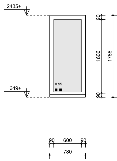
merk B2H als geteind: 2x geproefde: -- materiaal: hout 90x14mm vulling: geventileerde beglazing opmerking: intraswerendklasse 2 (NEN 5086)
