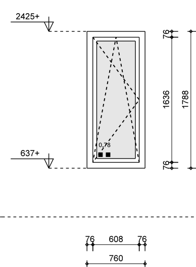
merk A1A als geteind: 2x geproefde: -- materiaal: aluminium vulling: geventileerde beglazing opmerking: intraswerendklasse 2 (NEN 5086)
