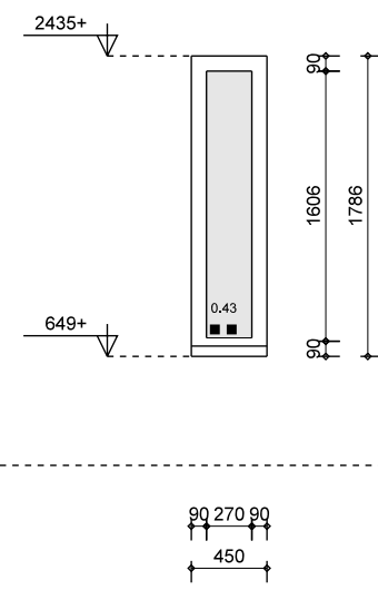
merk C1H als geteind: 1x geproefde: -- materiaal: hout 90x14mm vulling: geventileerde beglazing opmerking: intraswerendklasse 2 (NEN 5086)
