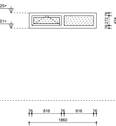
merk H1A als geteind: 1x geproefde: 1x materiaal: aluminium vulling: ondoorzichtige beglazing opmerking: intraswerendklasse 2 (NEN 5086)
