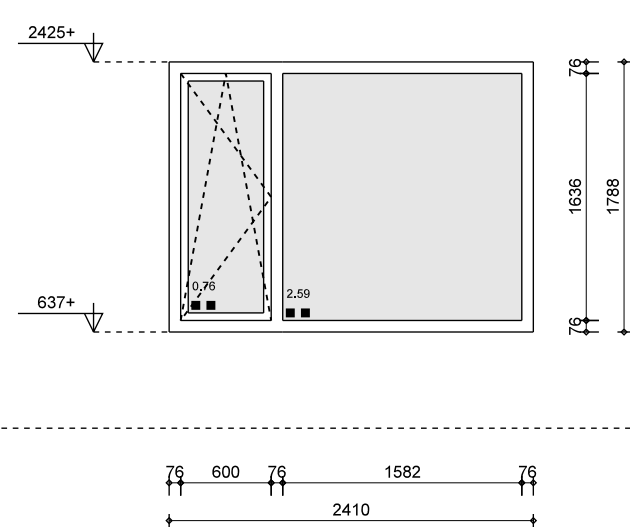
merk E1A als geteind: 2x geproefde: -- materiaal: aluminium vulling: geventileerde beglazing opmerking: intraswerendklasse 2 (NEN 5086)
