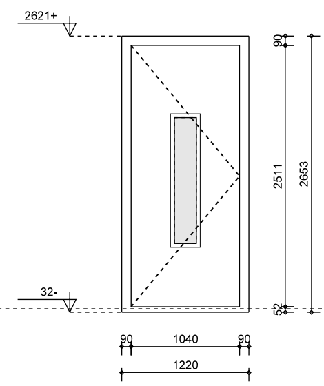
merk G1H als geteind: 1x geproefde: 1x materiaal: hout 90x14mm vulling: geventileerde aluina donce deur met glasstrook deur: Hübner Phoenix laag reflecterend opmerking: intraswerendklasse 2 (NEN 5086)
