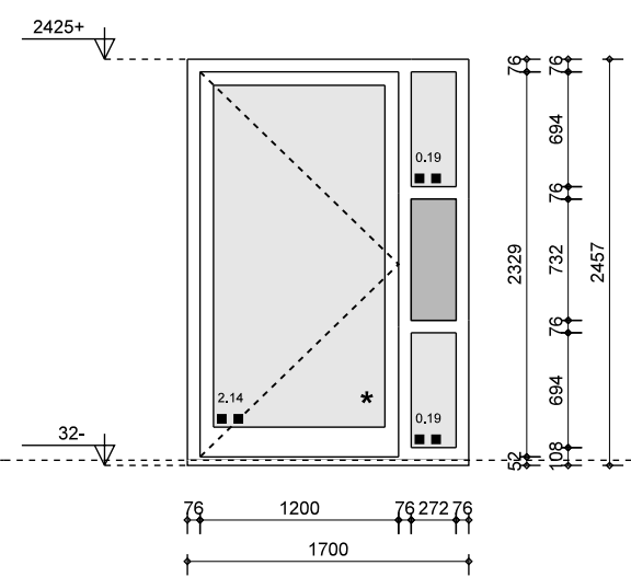
merk G1A als geteind: 1x geproefde: -- materiaal: aluminium vulling: geventileerde beglazing deur: paneel 1,3 x, hangopbouw aluminium deur x, x, geventileerde veiligheidsbeglazing (*) deur: Hübner Phoenix laag reflecterend opmerking: intraswerendklasse 2 (NEN 5086)
