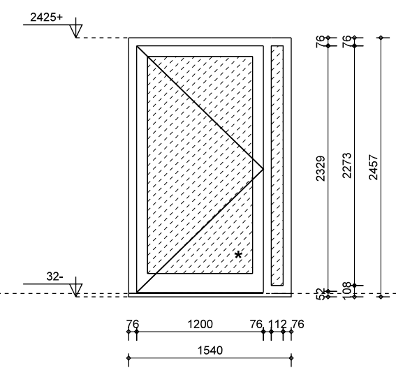
merk K1A als geteind: 1x (30 min VDBCO) geproefde: 1x materiaal: aluminium vulling: ondoorzichtige beglazing (1x 30 min VDBCO) deur: aluminium deur x, x, ondoorzichtige veiligheidsbeglazing (*) (1x 30 min VDBCO) deur: Hübner Phoenix laag reflecterend opmerking: intraswerendklasse 2 (NEN 5086)
