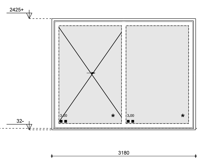
merk C1A als geteind: 2x geproefde: 2x materiaal: aluminium deur: schuifdeur 1x vast / 1x schuifend deel vulling: x, x, geventileerde veiligheidsbeglazing (*) deur: Hübner Phoenix laag reflecterend opmerking: intraswerendklasse 2 (NEN 5086)
