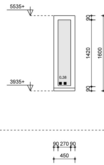
merk F1H als geteind: 1x geproefde: -- materiaal: hout 90x14mm vulling: geventileerde beglazing opmerking: intraswerendklasse 2 (NEN 5086)
