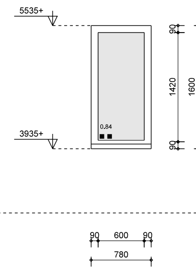
merk E2H als geteind: 2x geproefde: -- materiaal: hout 90x14mm vulling: geventileerde beglazing opmerking: intraswerendklasse 2 (NEN 5086)
