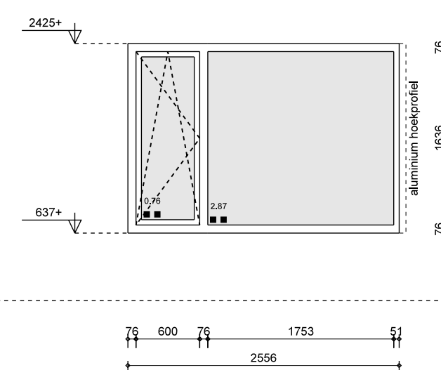
merk E2A als geteind: 1x geproefde: 1x materiaal: aluminium vulling: geventileerde beglazing opmerking: koppeling met aluminium hoekprofiel intraswerendklasse 2 (NEN 5086)
