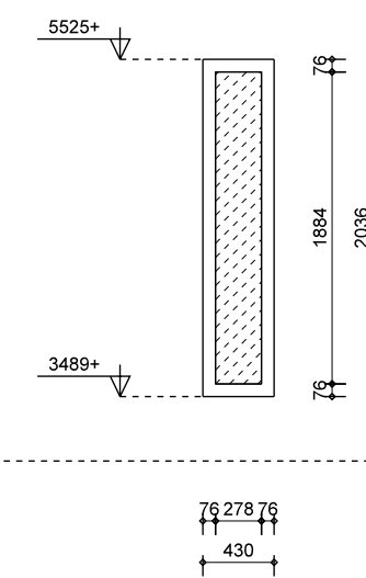
merk M1A als geteind: 7x geproefde: -- materiaal: aluminium vulling: aluminium opmerking: ondoorzichtige beglazing
