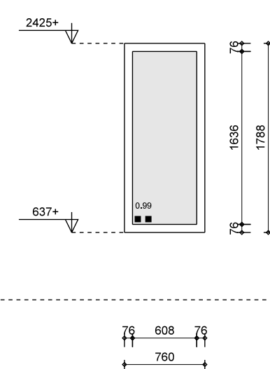
merk A2A als geteind: 2x geproefde: -- materiaal: aluminium vulling: geventileerde beglazing opmerking: intraswerendklasse 2 (NEN 5086)
