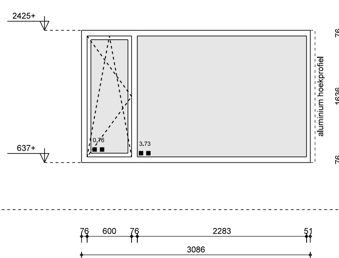
merk B2A als geteind: 1x geproefde: -- materiaal: aluminium vulling: geventileerde beglazing opmerking: koppeling met aluminium hoekprofiel intraswerendklasse 2 (NEN 5086)
