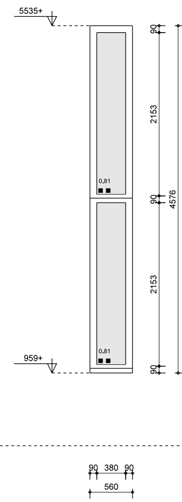
merk H1H als geteind: 1x geproefde: -- materiaal: hout 90x14mm vulling: geventileerde beglazing opmerking: intraswerendklasse 2 (NEN 5086)
