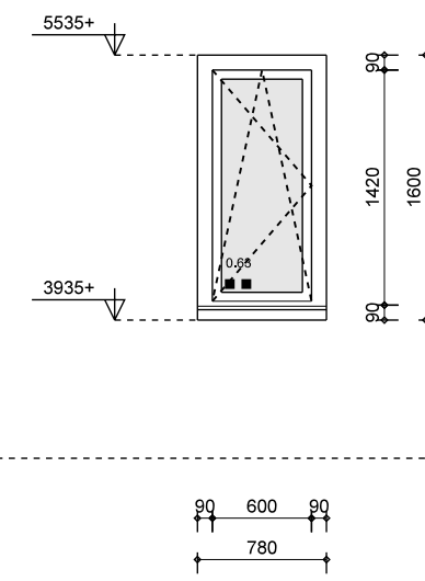
merk E1H als geteind: 1x geproefde: 1x materiaal: hout 90x14mm vulling: geventileerde beglazing opmerking: intraswerendklasse 2 (NEN 5086)
