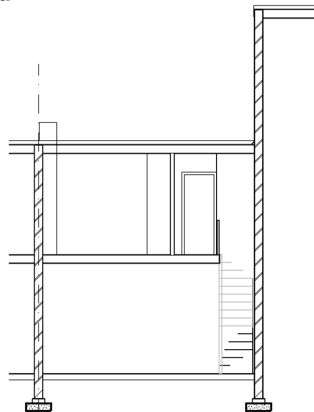
Doorsnede B-B bestand
