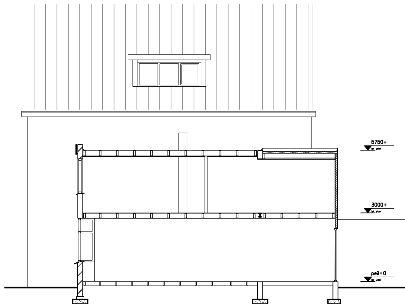
Doorsnede A-A bestand
