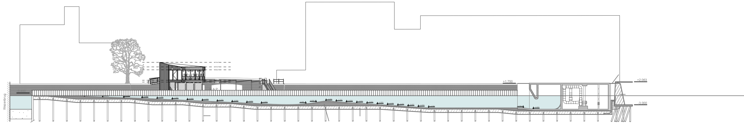
DOORSNEDE A-A SCHAAL 1:200
