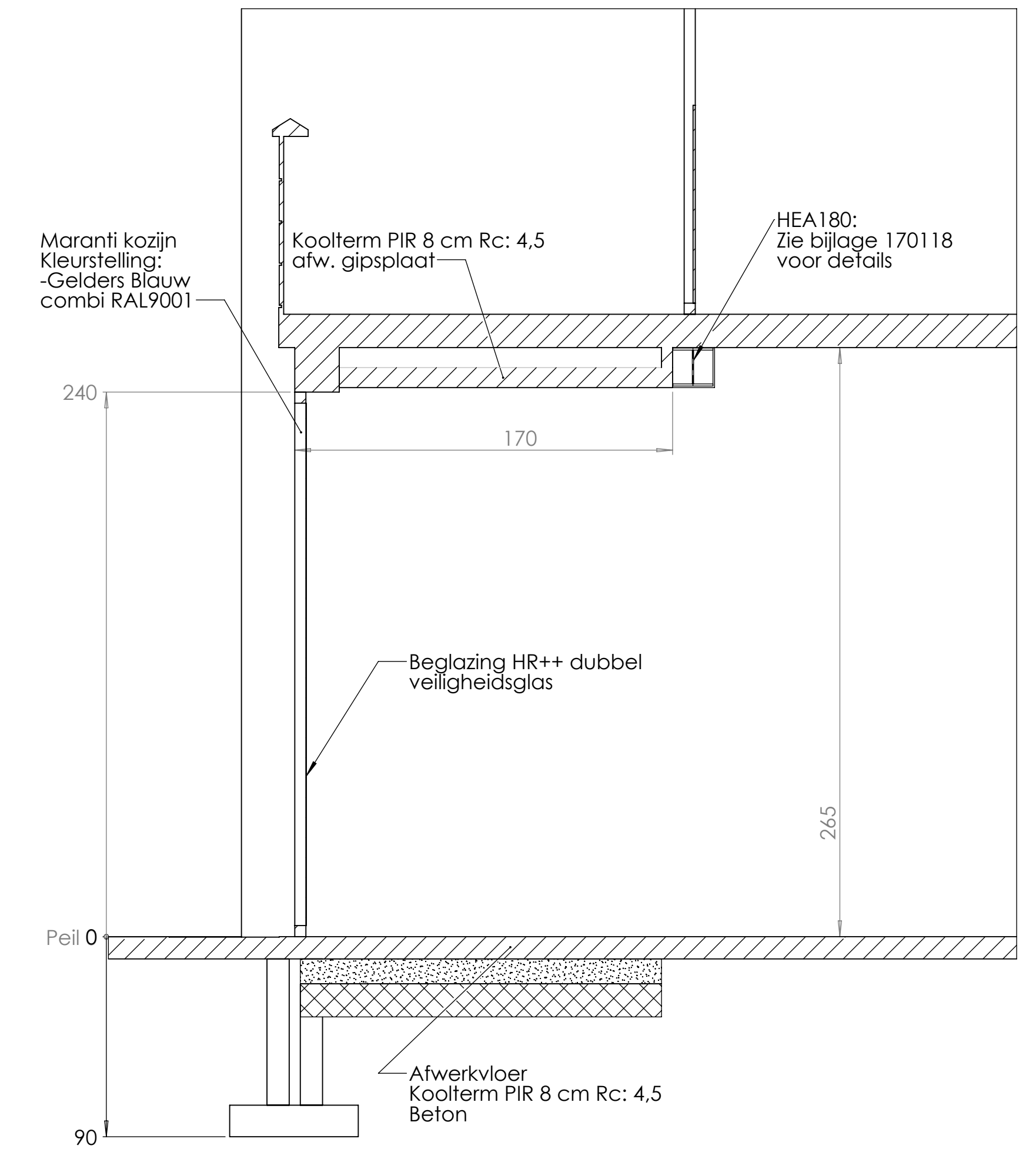
SECTION A-A SCHAAL 1 : 20
