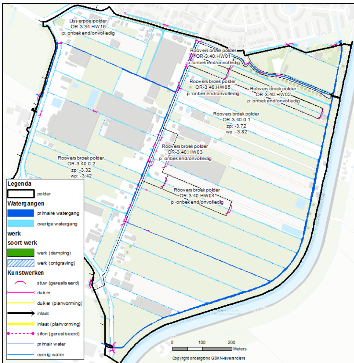
Figuur 3-12 Watersysteem Rooversbroekpolder
