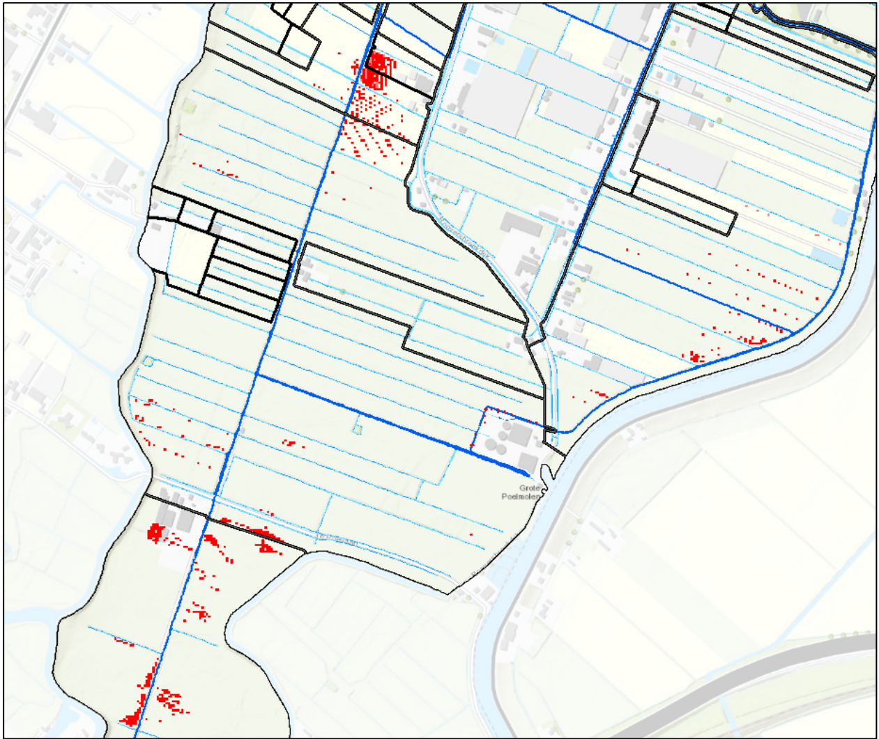
Figuur 4-2 Inundatiekaart van de Lisserpolder en Rooversbroekpolder
