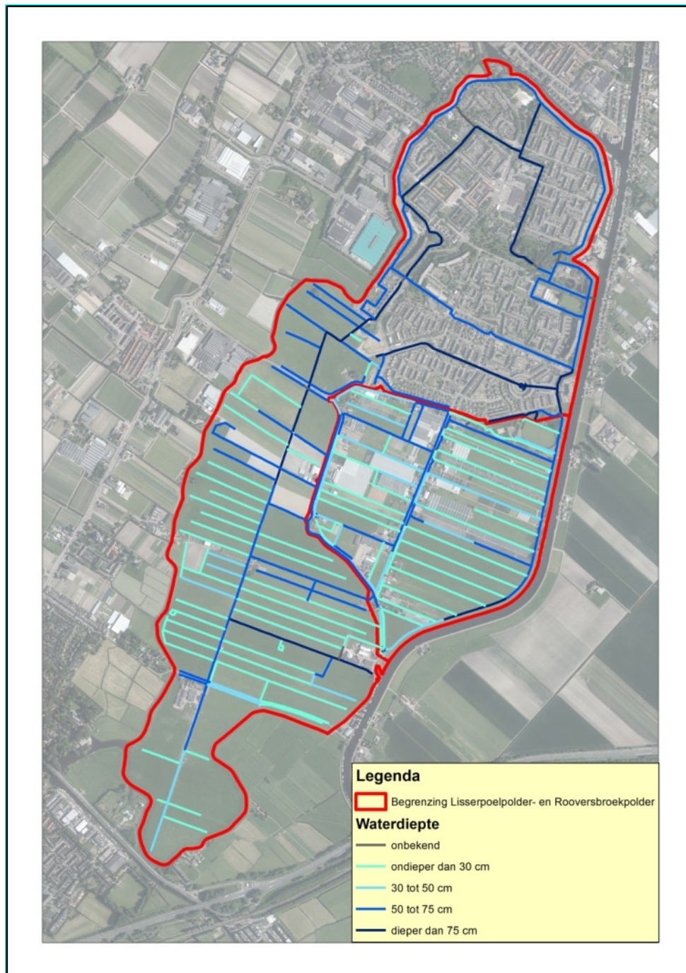
Figuur 3-14 Diepte van de watergangen in het plangebied
