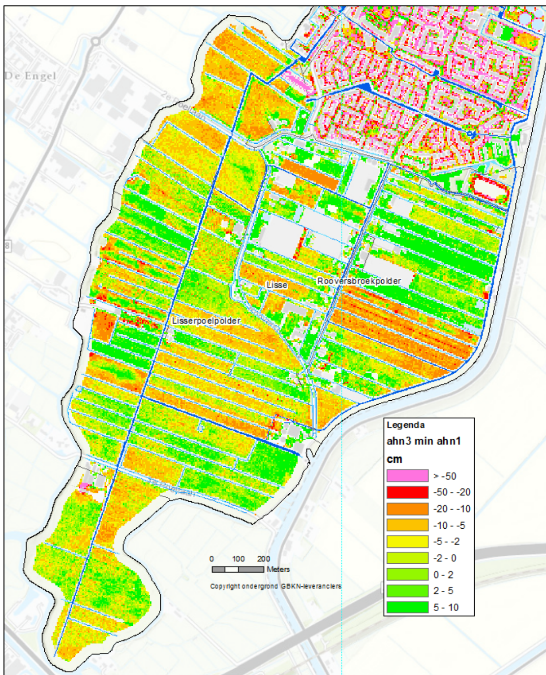
Figuur 3-7 Maaiveldhoogteverschil tussen 2014 en 2003
