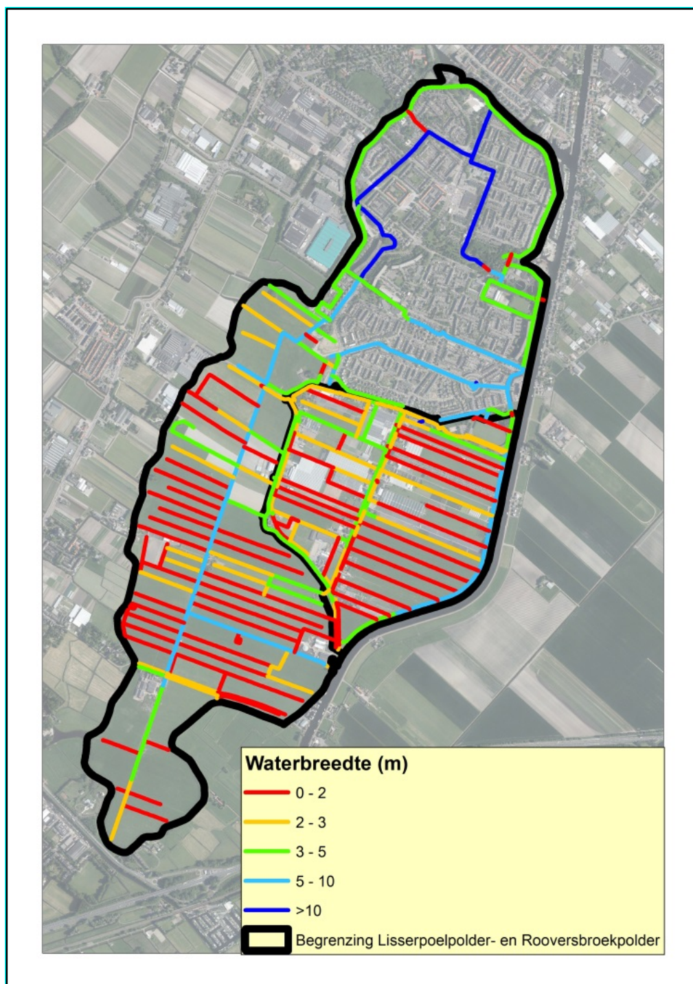
Figuur 3-16 Breedte watergangen op waterlijn
