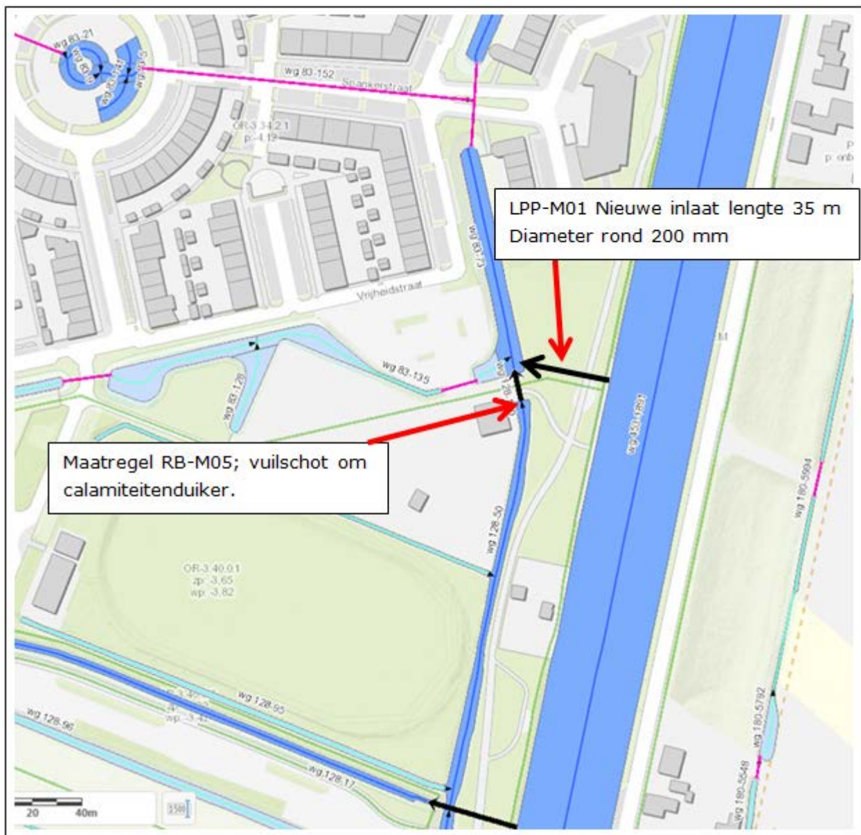
Figuur 5-3 Maatregelen RB-M05 en LPP-M01
