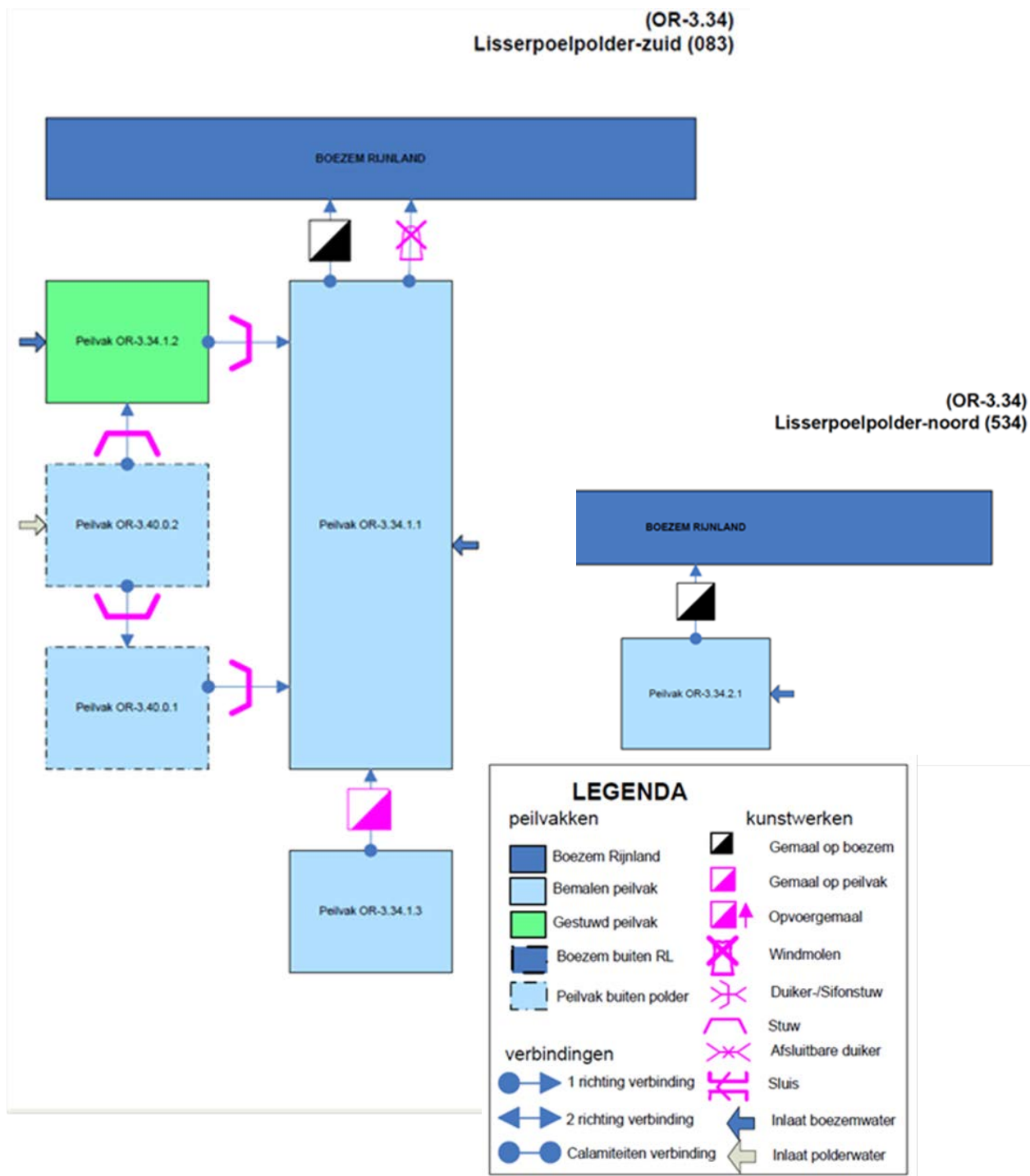
Figuur 3-13 Theoretisch aan- en afvoerschema peilvakken Lisserpoelpolder en Rooversbroekpolder
