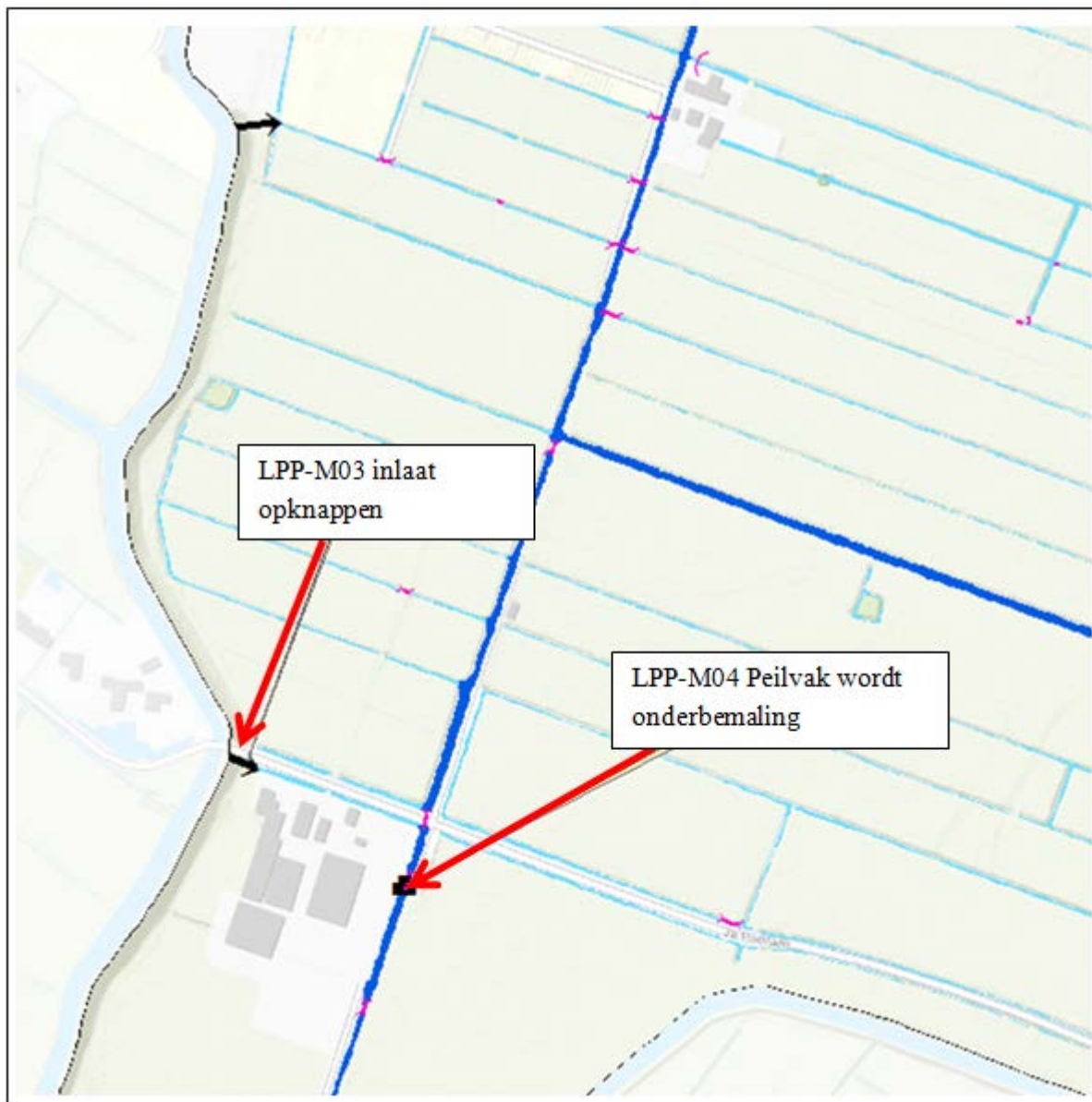
Figuur 5-6 Maatregel LPP-M03 en LPP-M04
