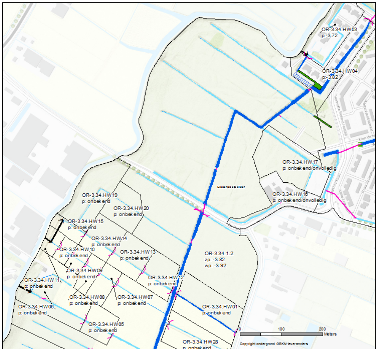
Figuur 3-10 Het watersysteem van het midden van de Lisserpoelpolder, met de vele hoogwaterzones.
