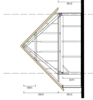
DOORSNEDE B-B
