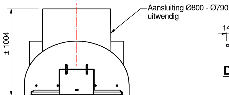
Bovenaanzicht
