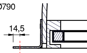
Doorsnede C-C
