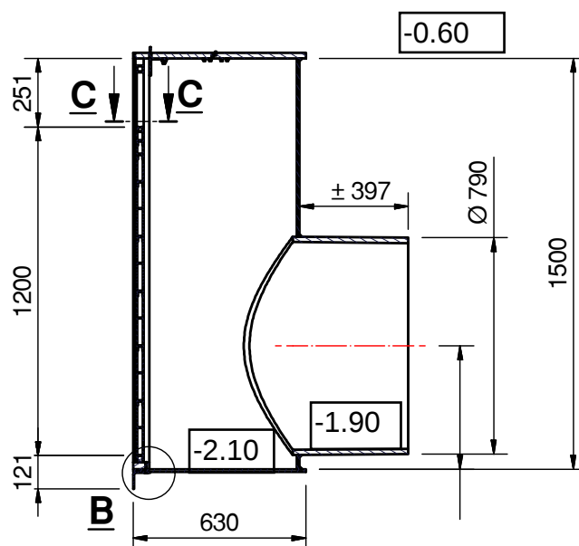
Doorsnede A-A
