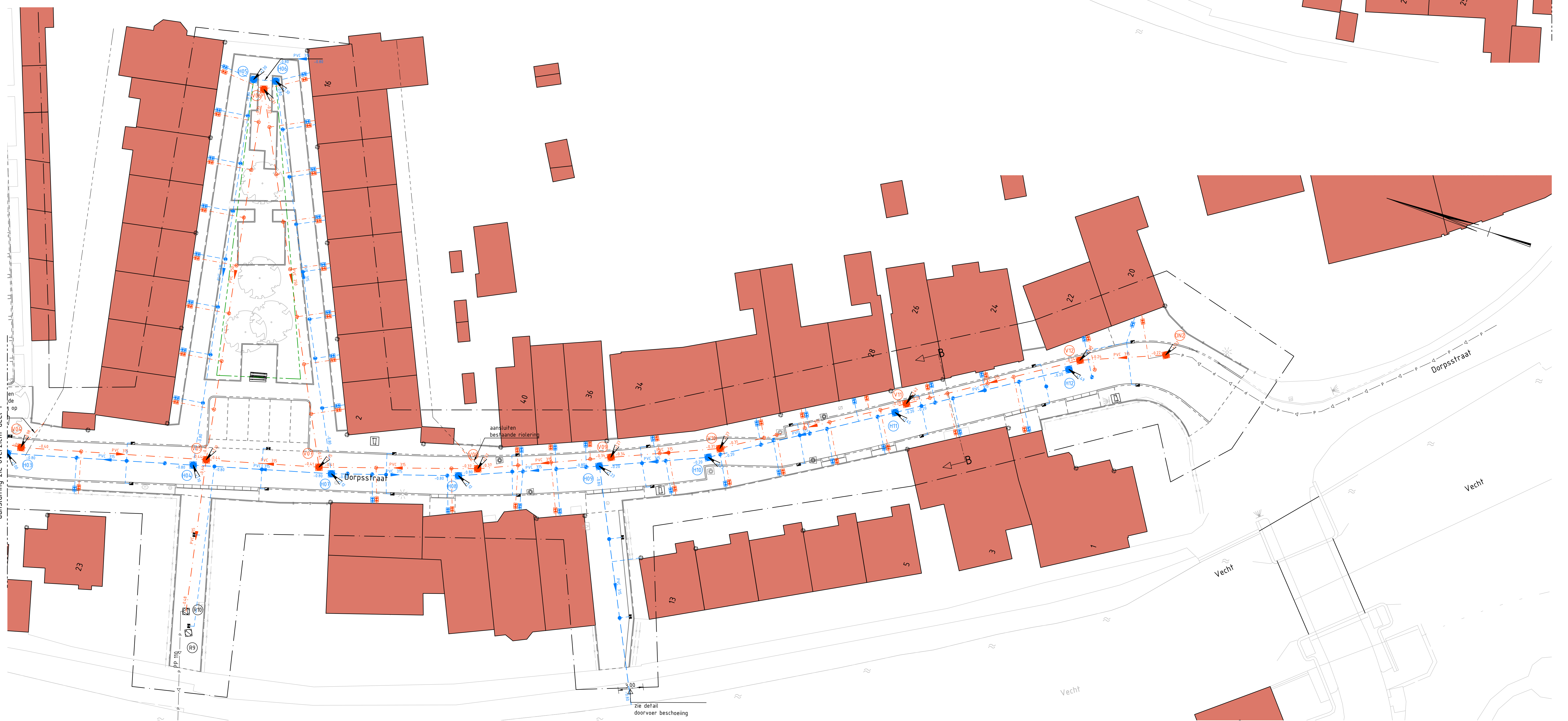
Overzicht situatie deel 2 SCHAAL 1 : 200
