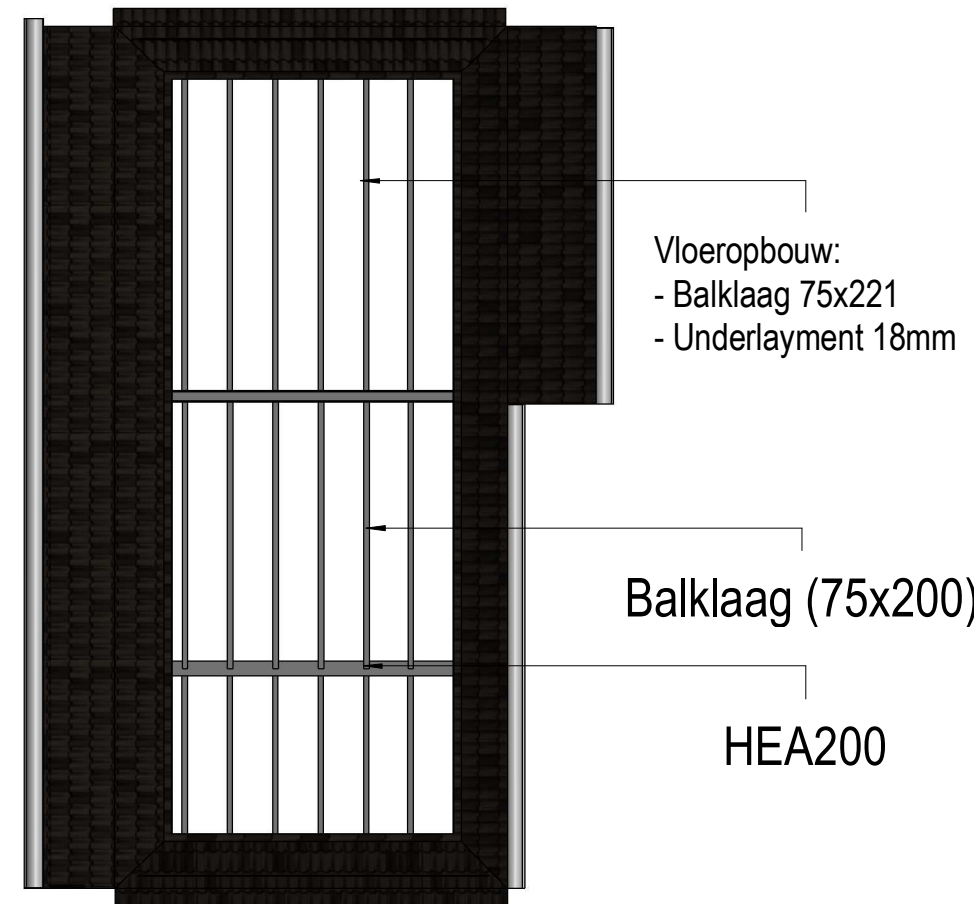
Constructieoverzicht
