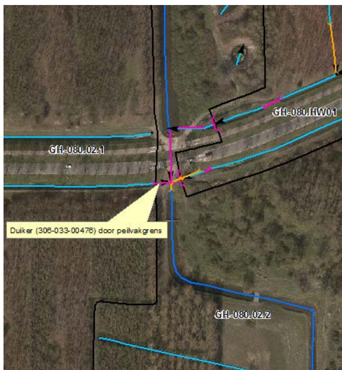
Figuur 5.2: Duiker door peilscheiding GH-080.02.1 en GH-080.02.2
