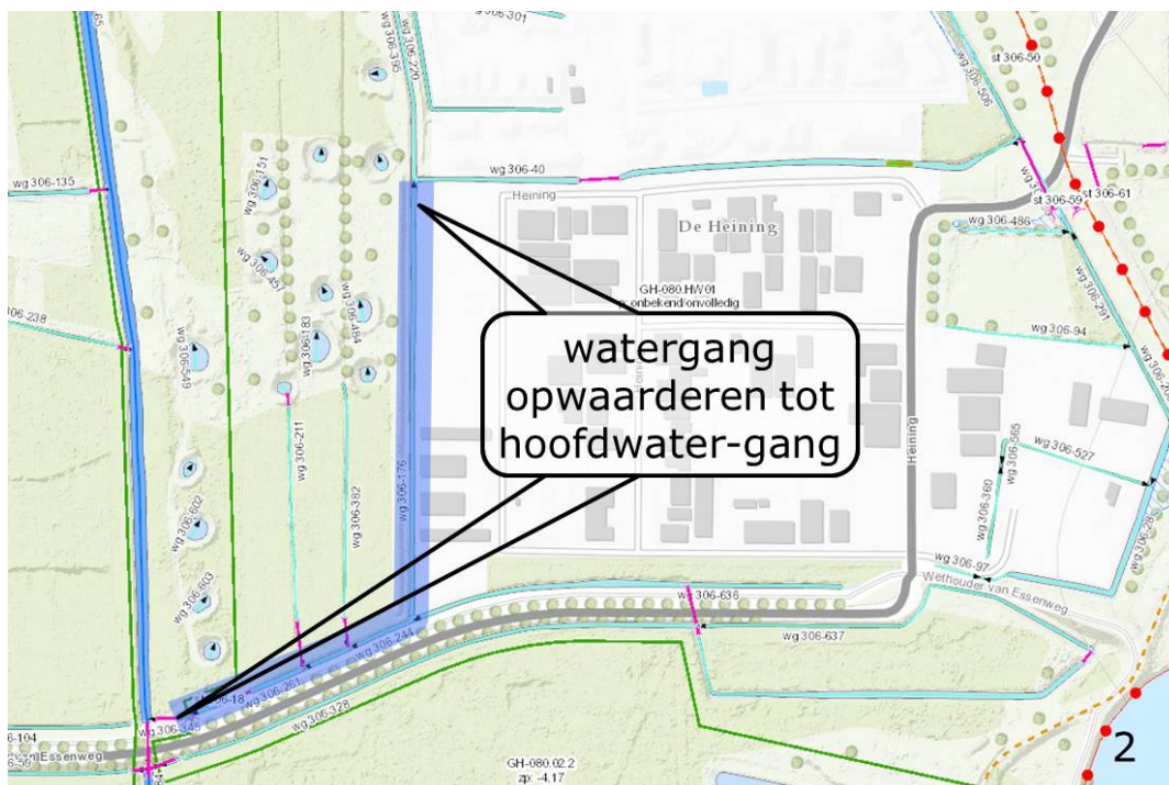
Figuur 6.7: Opwaarderen tot hoofdwatergang Heining
