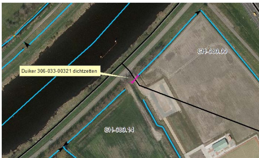
Figuur 6.6: Dichtzetten duiker
