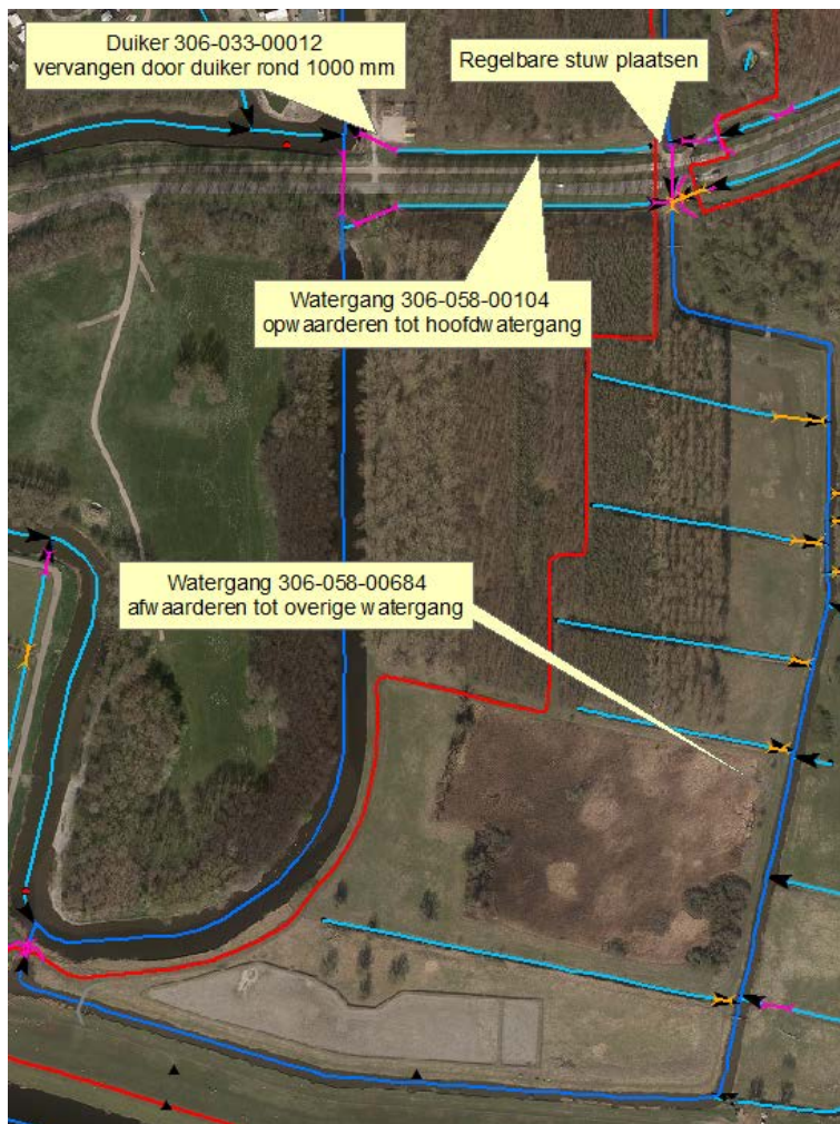
Figuur 6.4: Aanpassen hoofdafvoer GH-080.02.2
