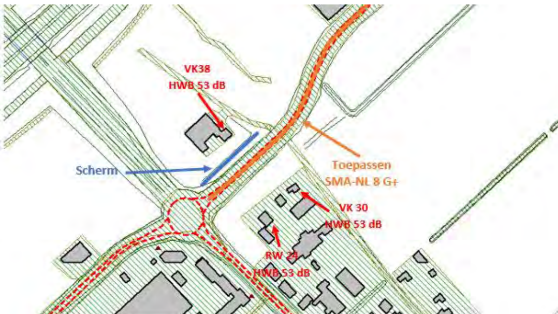
Figuur 4.4. Maatregelen en benodigde hogere waarden a.g.v. reconstructie Duurzaamheidstraat
