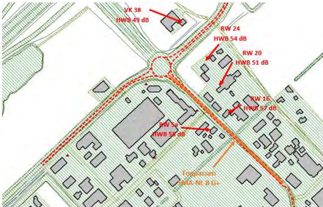
Figuur 4.3. Maatregelen en benodigde hogere waarden a.g.v. reconstructie Rondweg
