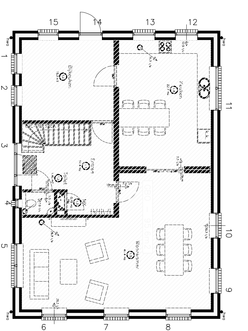
Begane grond Woonfunctie: Gebruiksoppervlakte begane grond
