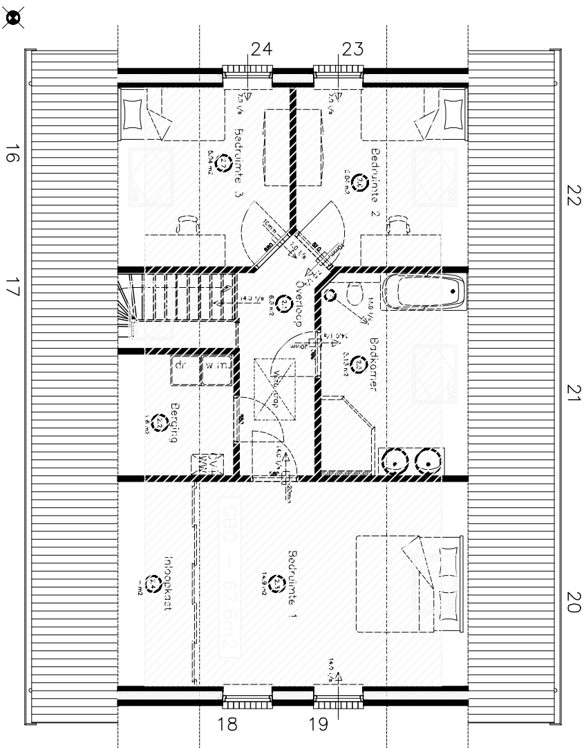
Verdieping Woonfunctie: Gebruiksoppervlakte verdieping
