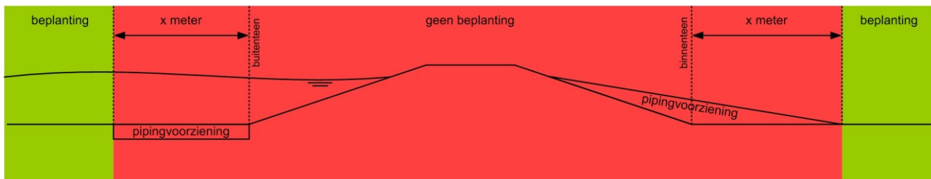
Figuur AR1.2: beplanting pipingvoorziening
