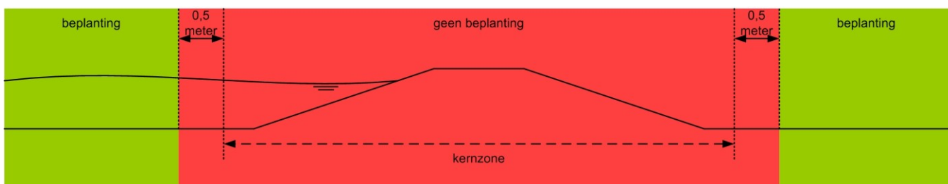
Figuur AR1.3: beplanting kadastrale erfafscheiding niet verheelde en niet aangeeelde waterkering
