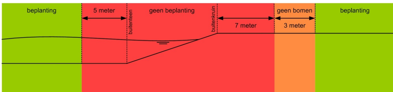
Figuur AR1.4: beplanting verheelde en aangeeelde waterkering
