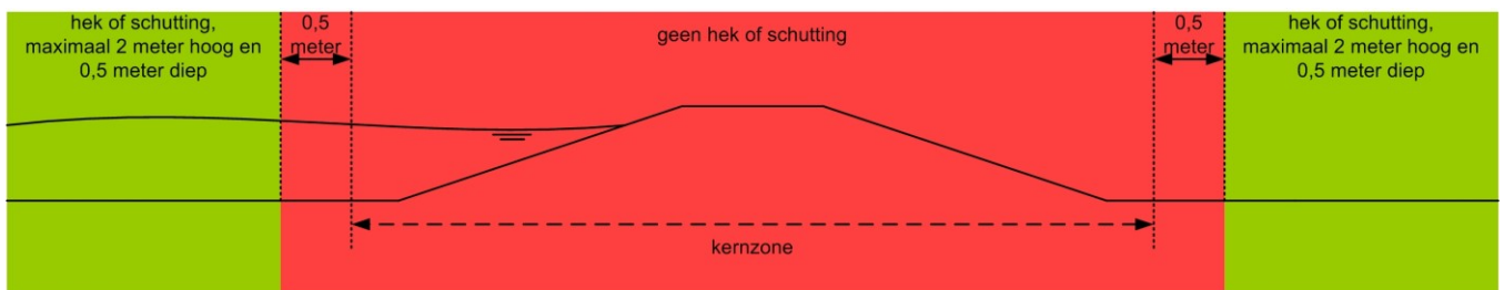
Figuur AR3.2: hek of schutting kadastrale erfafscheiding niet verheelde en niet aangeheelde waterkering
