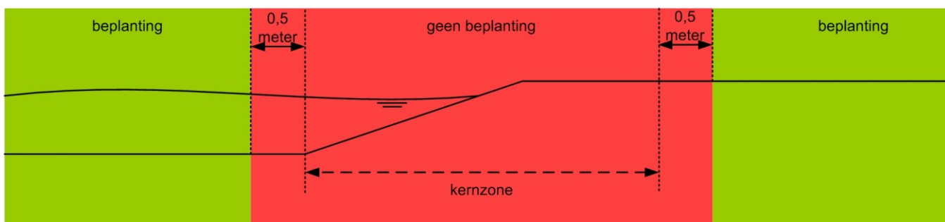
Figuur AR1.5: beplanting kadastrale erfafscheiding verheelde en aangeeelde waterkering
