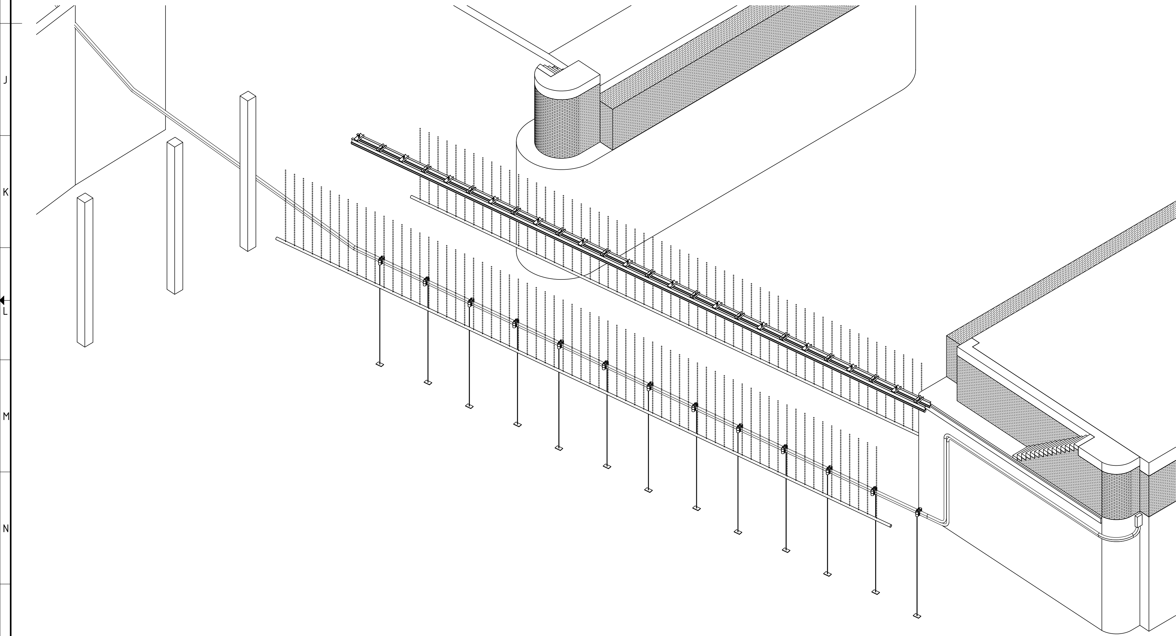
3D ZINKER MET TIJDELIJKE VOORZIENINGEN
