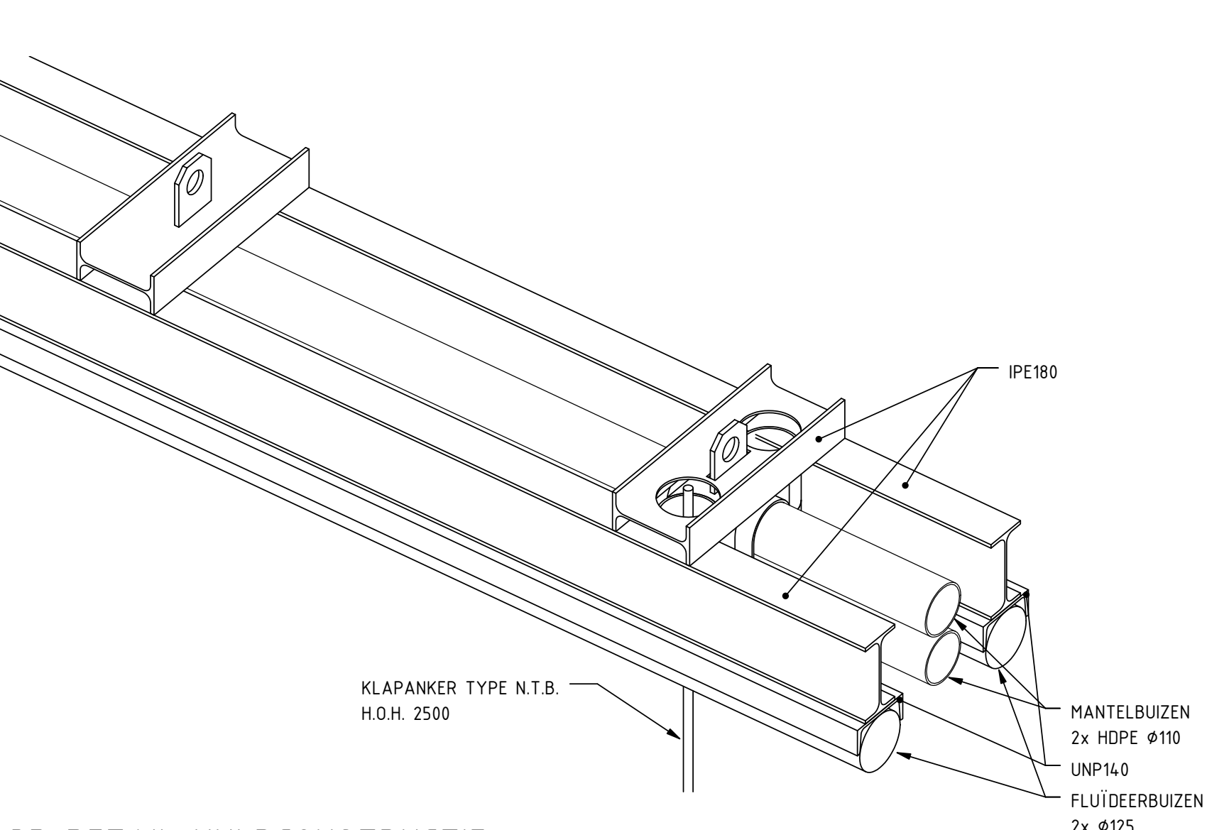
3D DETAIL HULPCONSTRUCTIE
