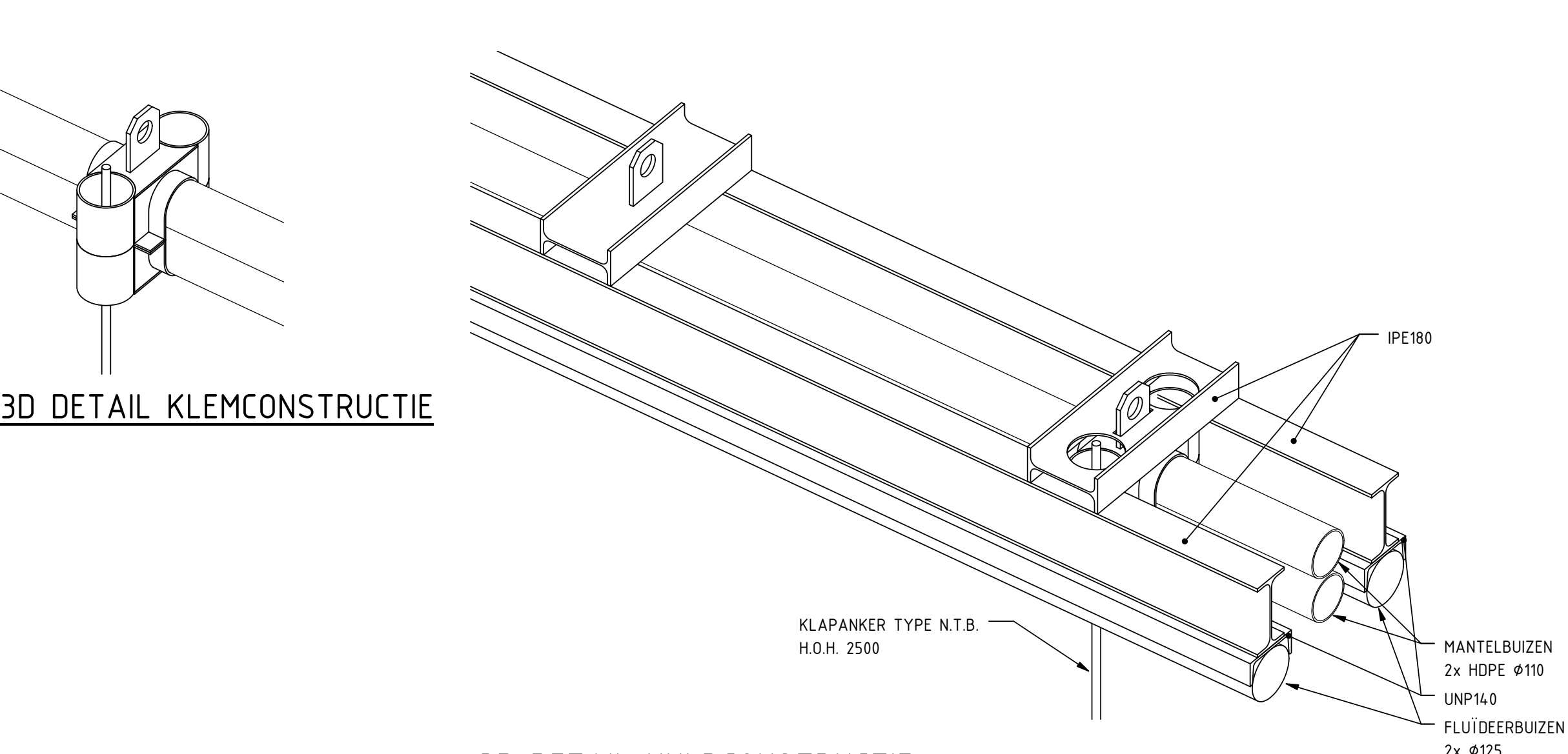
3D DETAIL HULPCONSTRUCTIE
