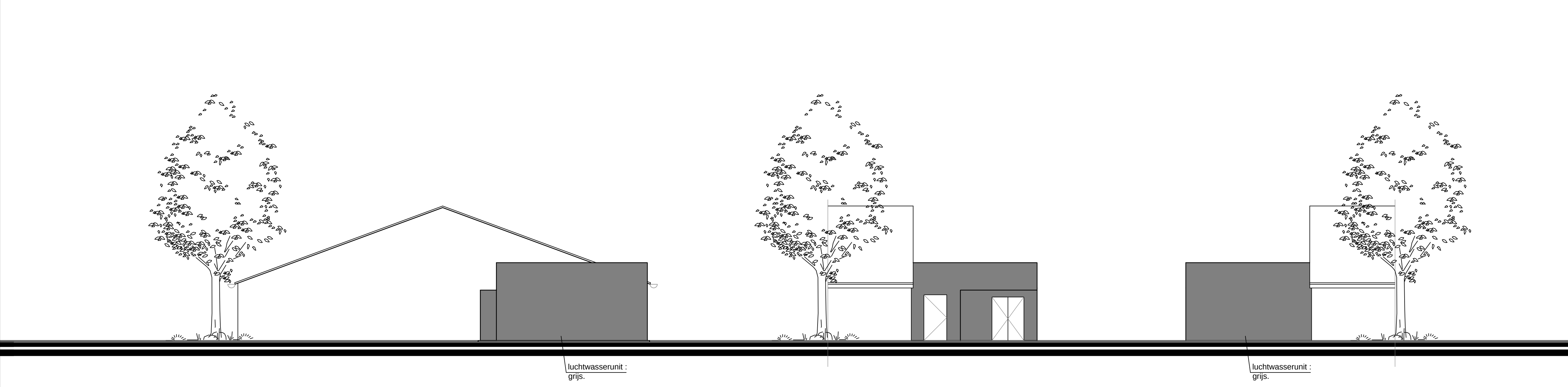
ACHTERAANZICHT ,EN ZIJAANZICHTEN, GEDEELTE BESTAANDE VARKENSSTAL , -1- , MET LUCHTWASSER
