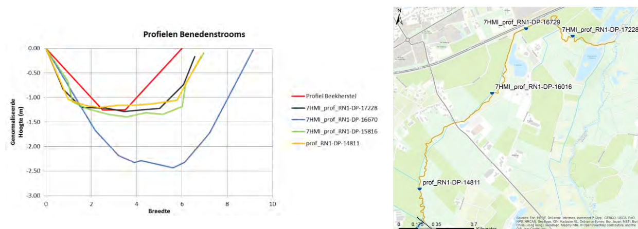
Figuur 3-7. Selectie bestaande profielen Benedenstrooms in relatie tot profiel beekherstel
