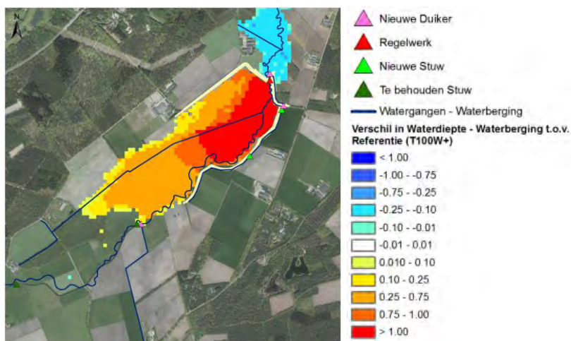
Figuur 4-4. Verschil in waterdiepte T100Wh Waterberging ten opzichte van de referentie.
