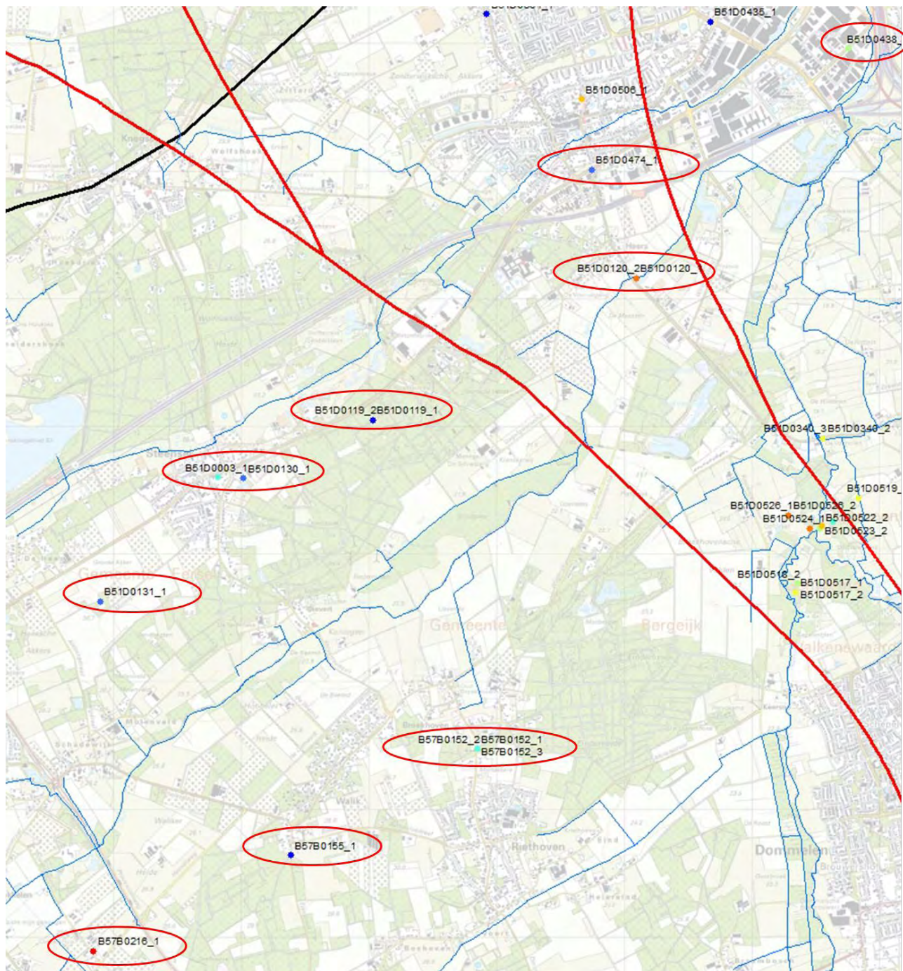
Figuur 14 Locatie peilbuizen die geschikt zijn voor directe vergelijking met modelresultaten.
