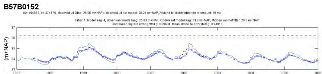
Figuur 20 Vergelijking meting (blauw) en berekening (groen) bij peilbuis B57B0152.
