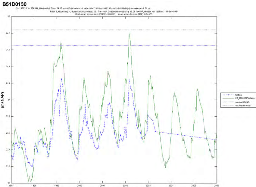
Figuur 22 Vergelijking meting (blauw) en berekening (groen) bij peilbuis B51D0130.
