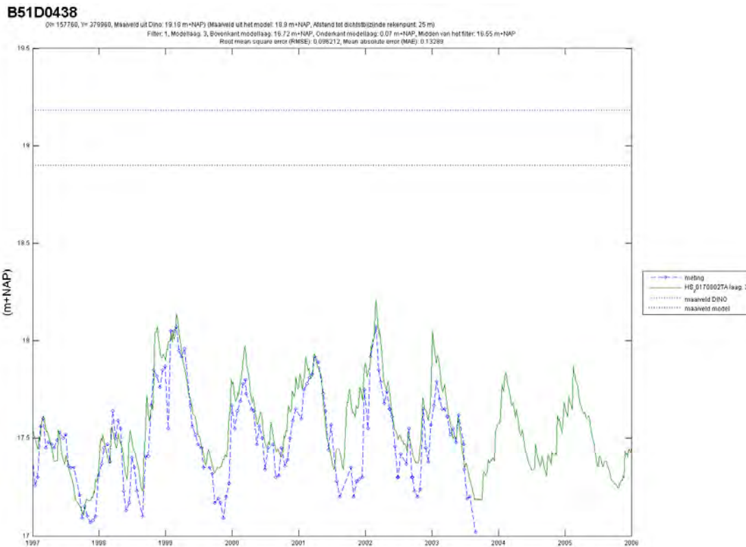
Figuur 26 Vergelijking meting (blauw) en berekening (groen) bij peilbuis B51D0438.
