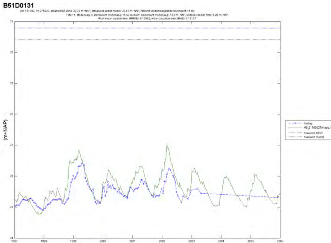
Figuur 19 Vergelijking meting (blauw) en berekening (groen) bij peilbuis B51D0131.
