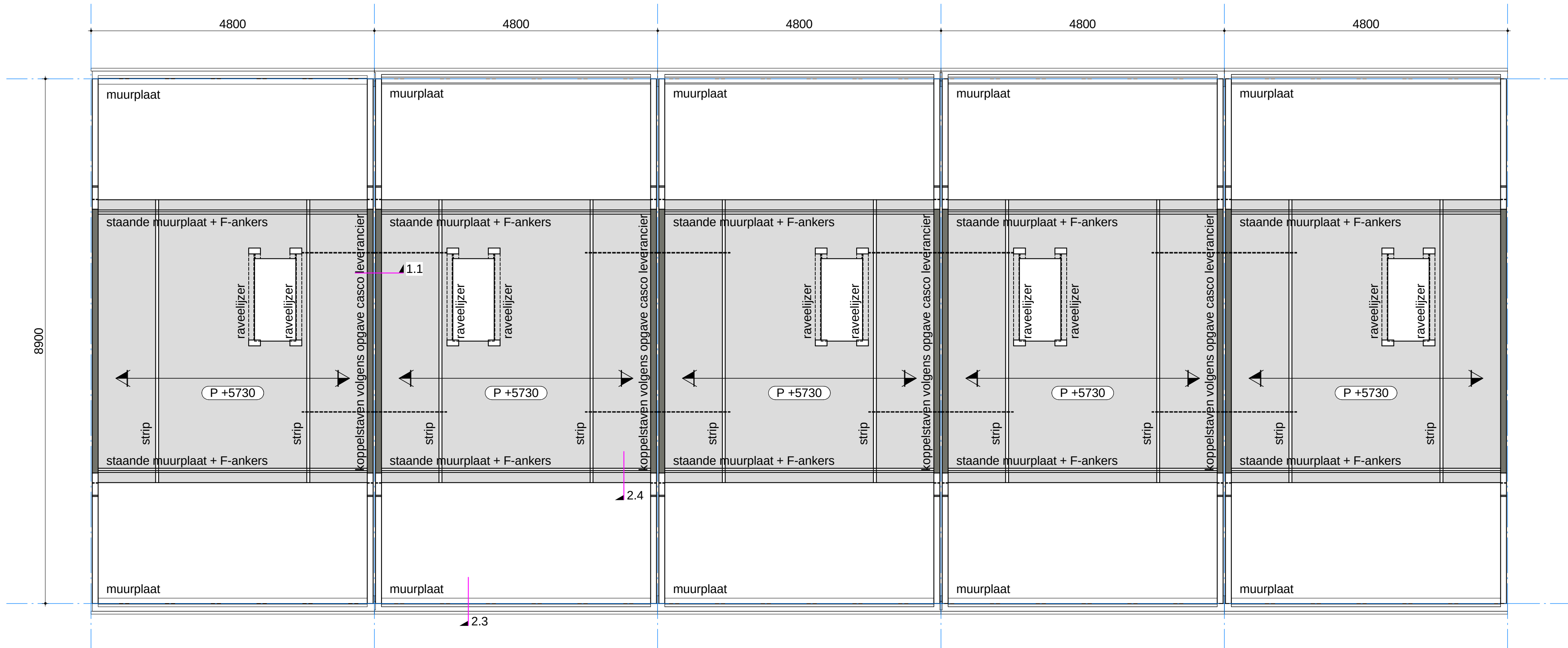
2e verdiepingsvloer muurplaat en F-anker volgens opgave kapleverancier strip t.b.v. spatkrachten kap en raveelijzer volgens opgave vloerenleverancier
