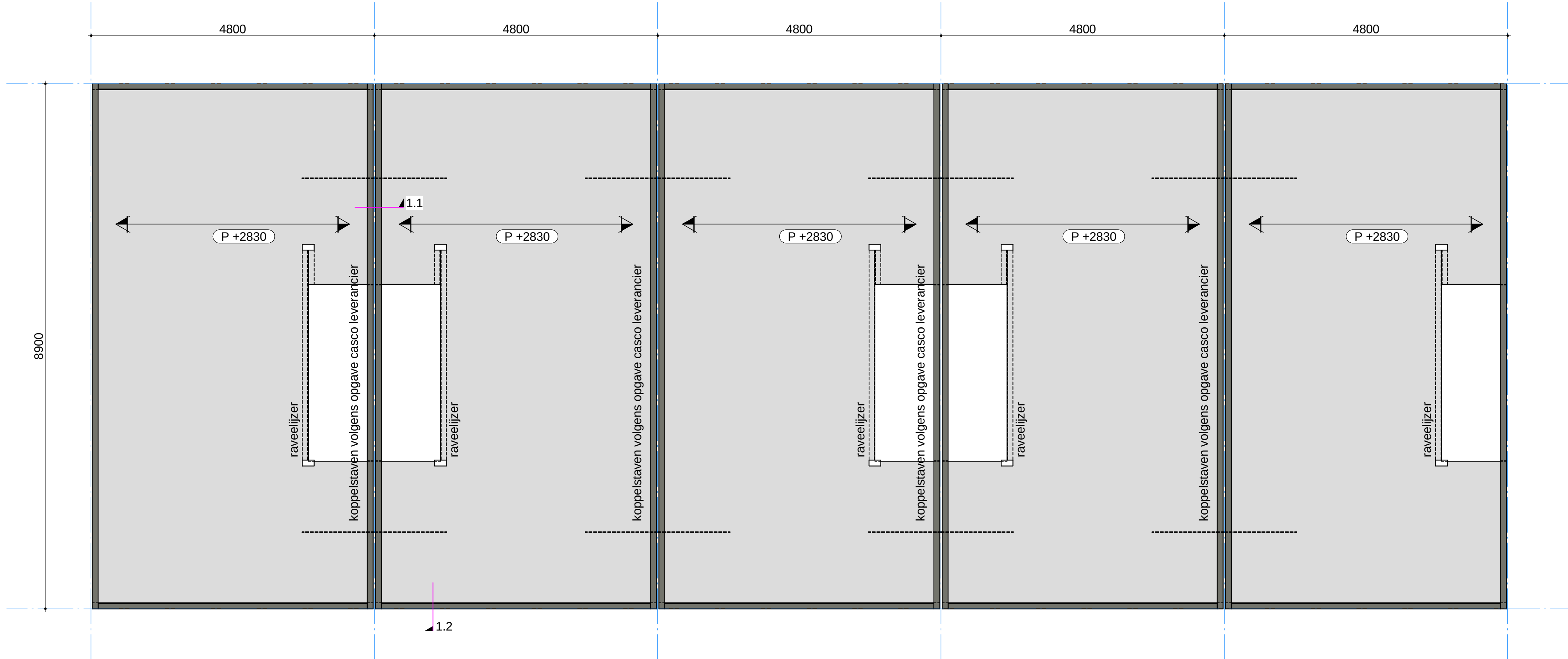
1e verdiepingsvloer raveelijzer volgens opgave vloerenleverancier
