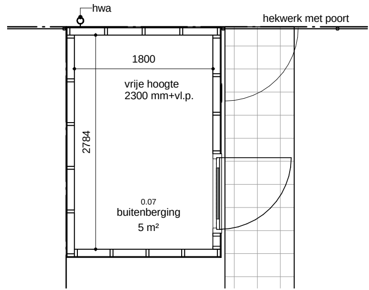
Berging enkel
