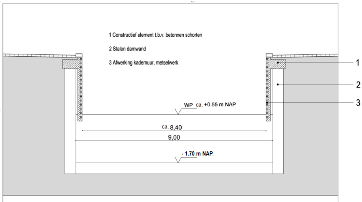
Figuur 6: principedoorssnede Roode Vaart tussen N285 en overkluizingsconstructie
