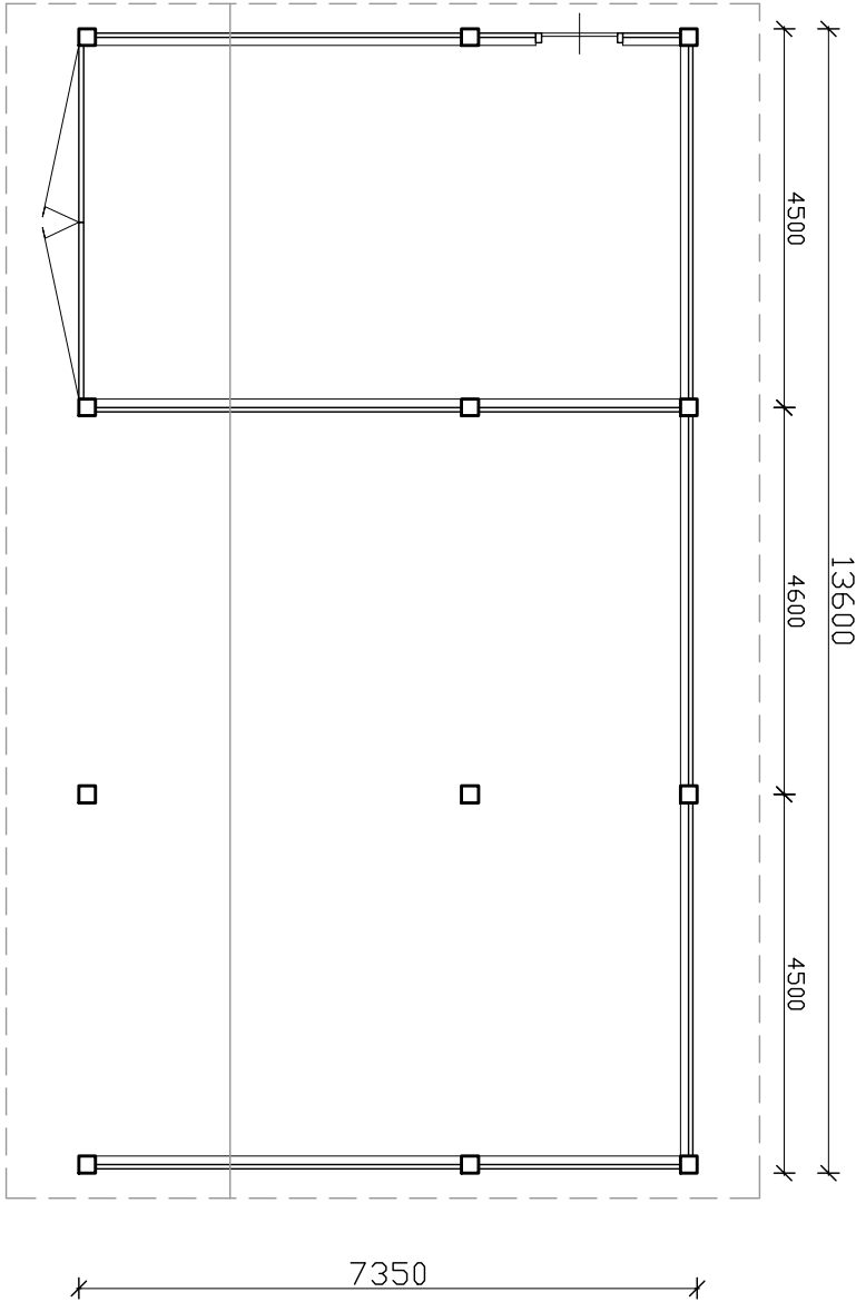
Bijgebouw (Kapschuur)
