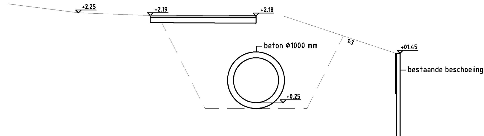
Dwarsprofiel F-F
