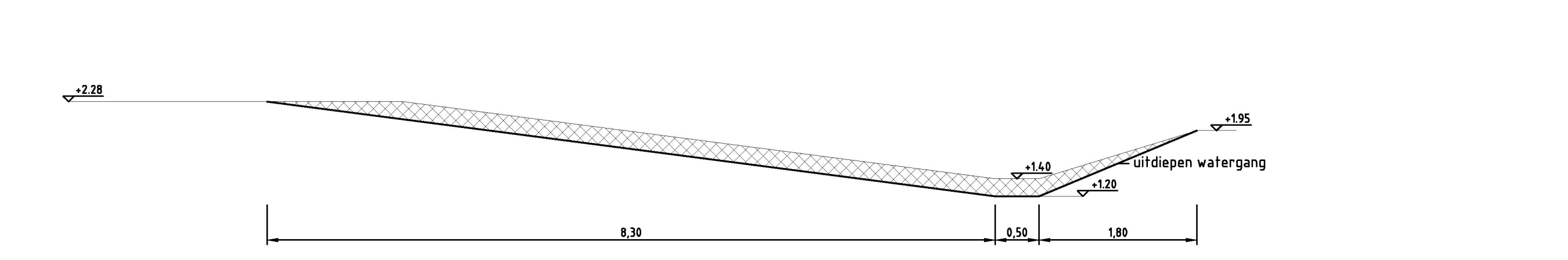
Dwarsprofiel D-D
