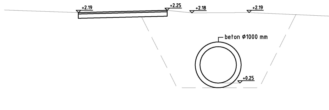
Dwarsprofiel G-G
