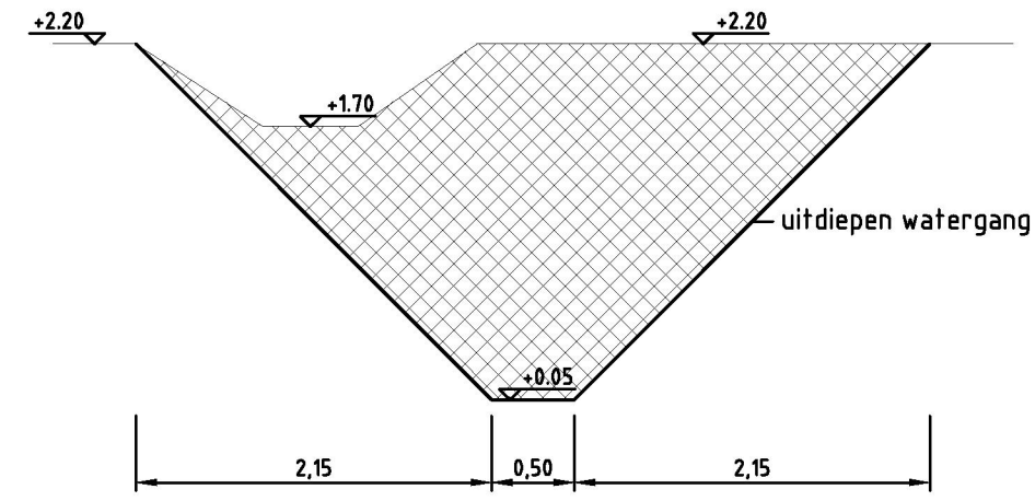
Dwarsprofiel H-H
