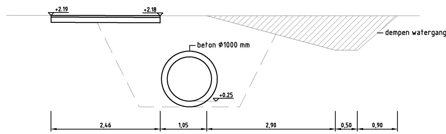
Dwarsprofiel E-E
