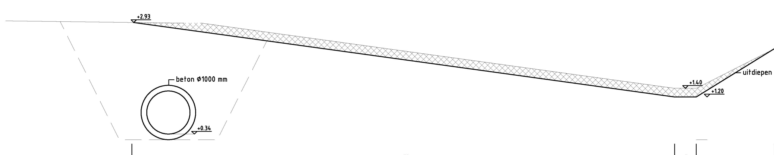
Dwarsprofiel C-C
