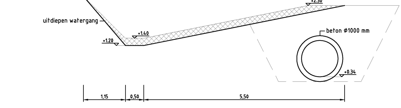
Dwarsprofiel B-B
