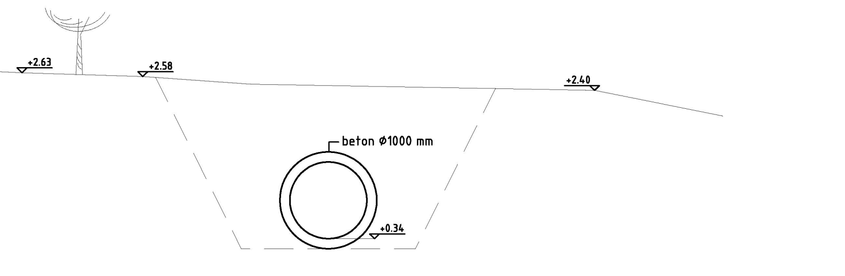
Dwarsprofiel A-A
