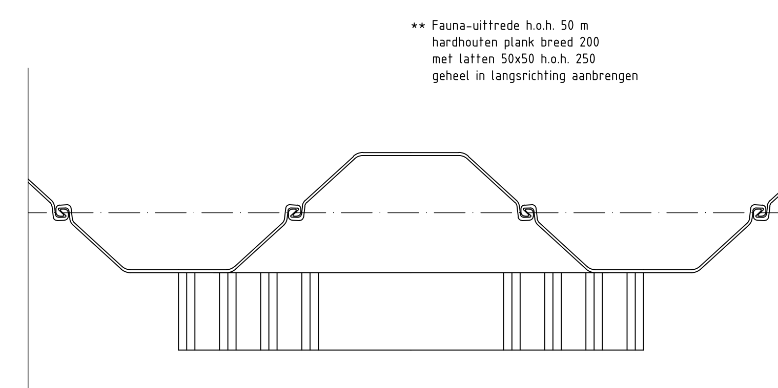
Bovenaanzichtl fauna uittrede SCHAAL 1:10
