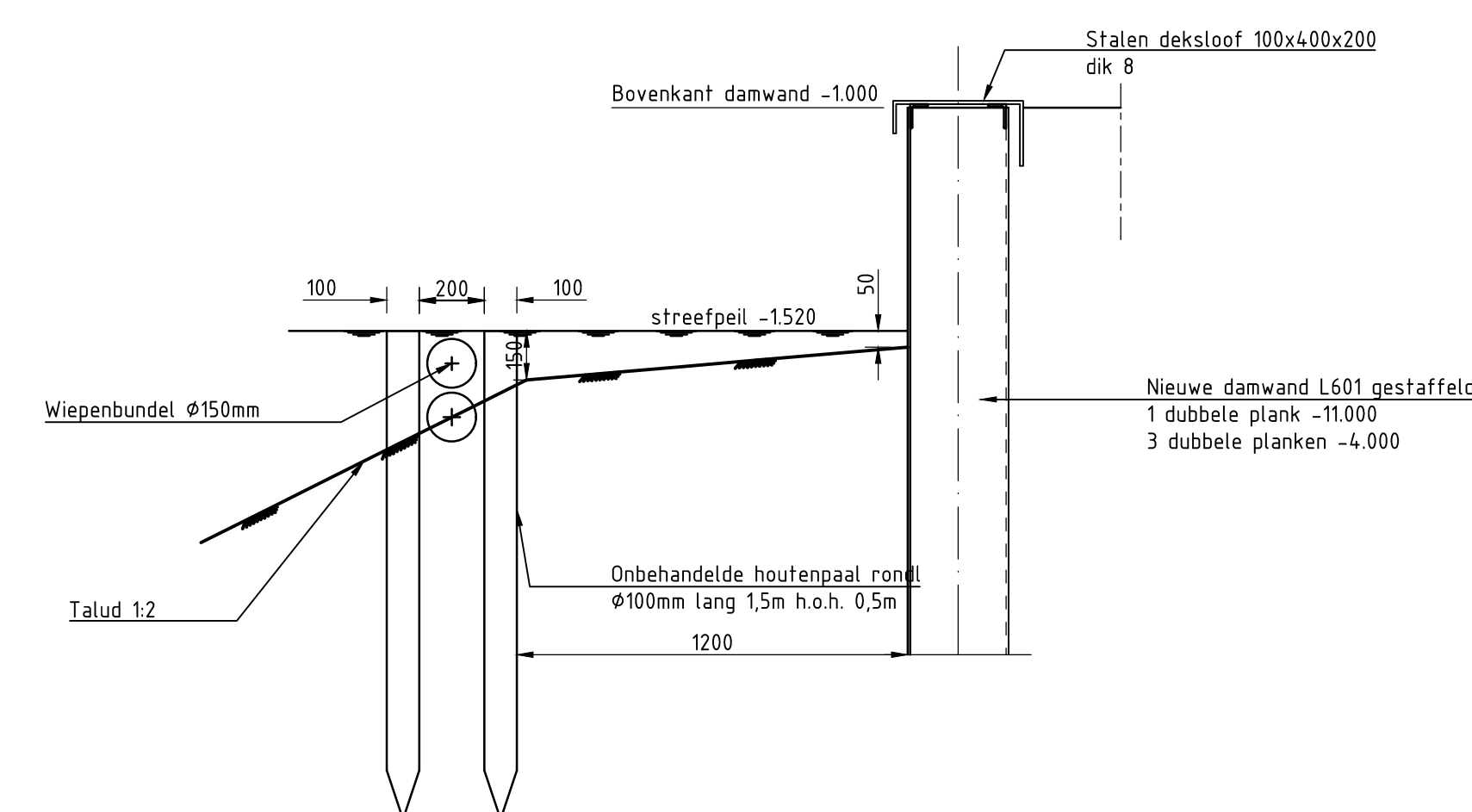
Detail t.p.v. Plasdraszone SCHAAL 1:20
