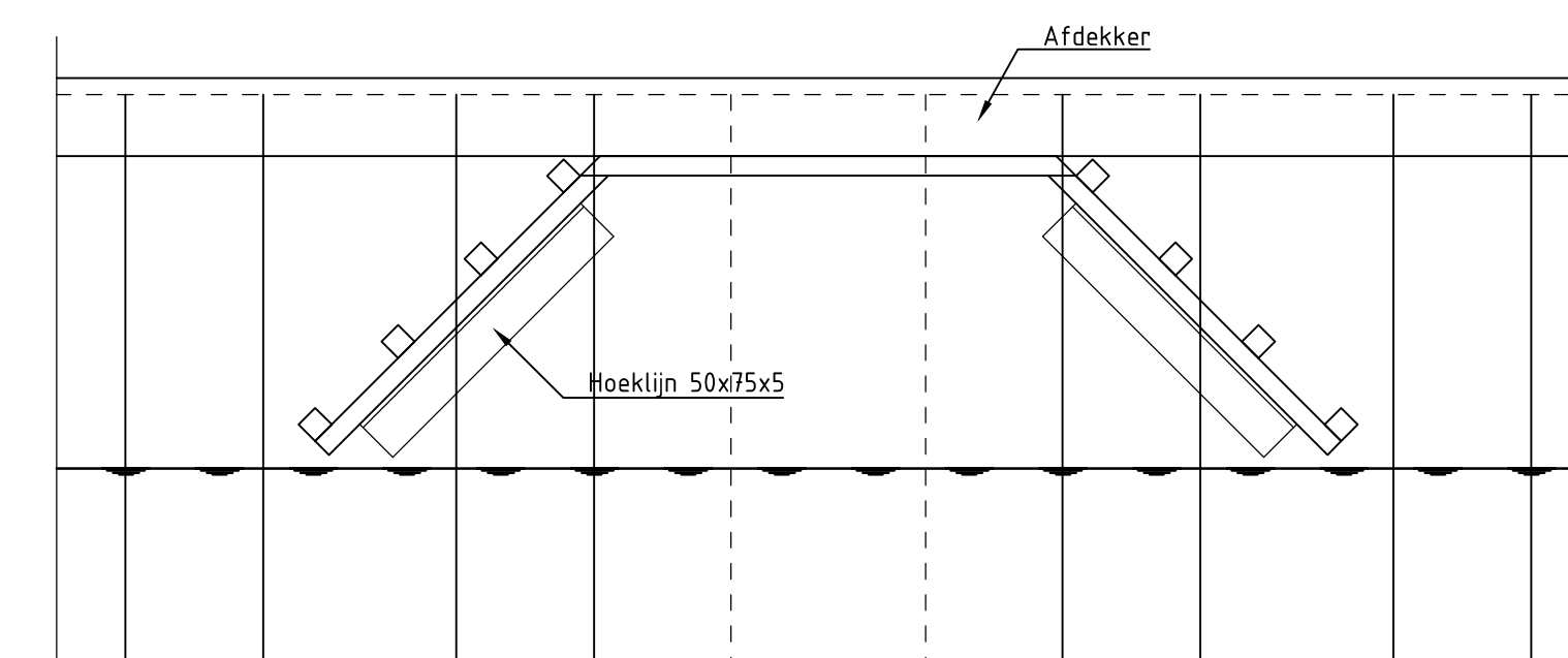
Aanzicht fauna uittrede SCHAAI 1:10
