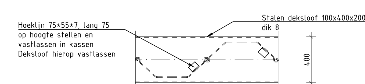
Principe bovenaanzicht deksloof SCHAAL 1:20
