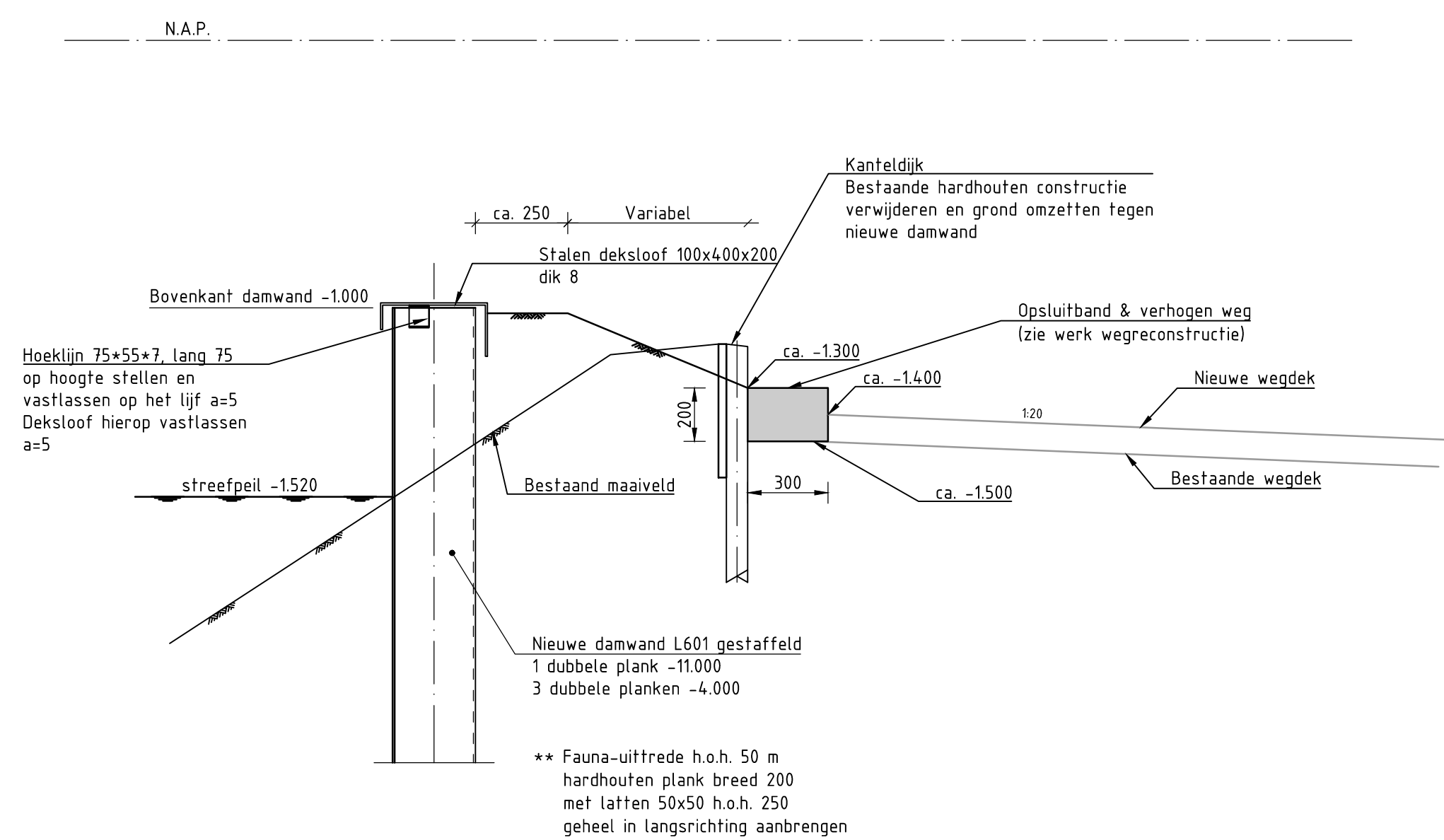
Principe doorsnede SCHAAL 1:20
