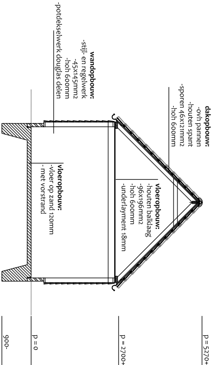
doorsnede tpv zoldervloer
