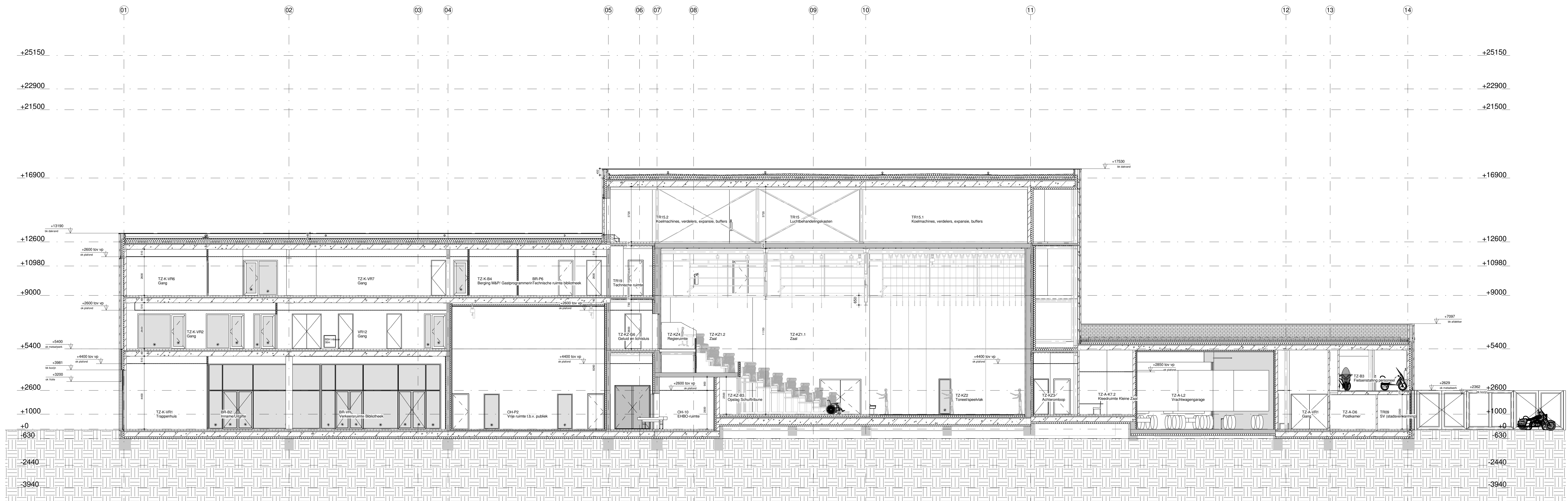
doorsnede A-A
