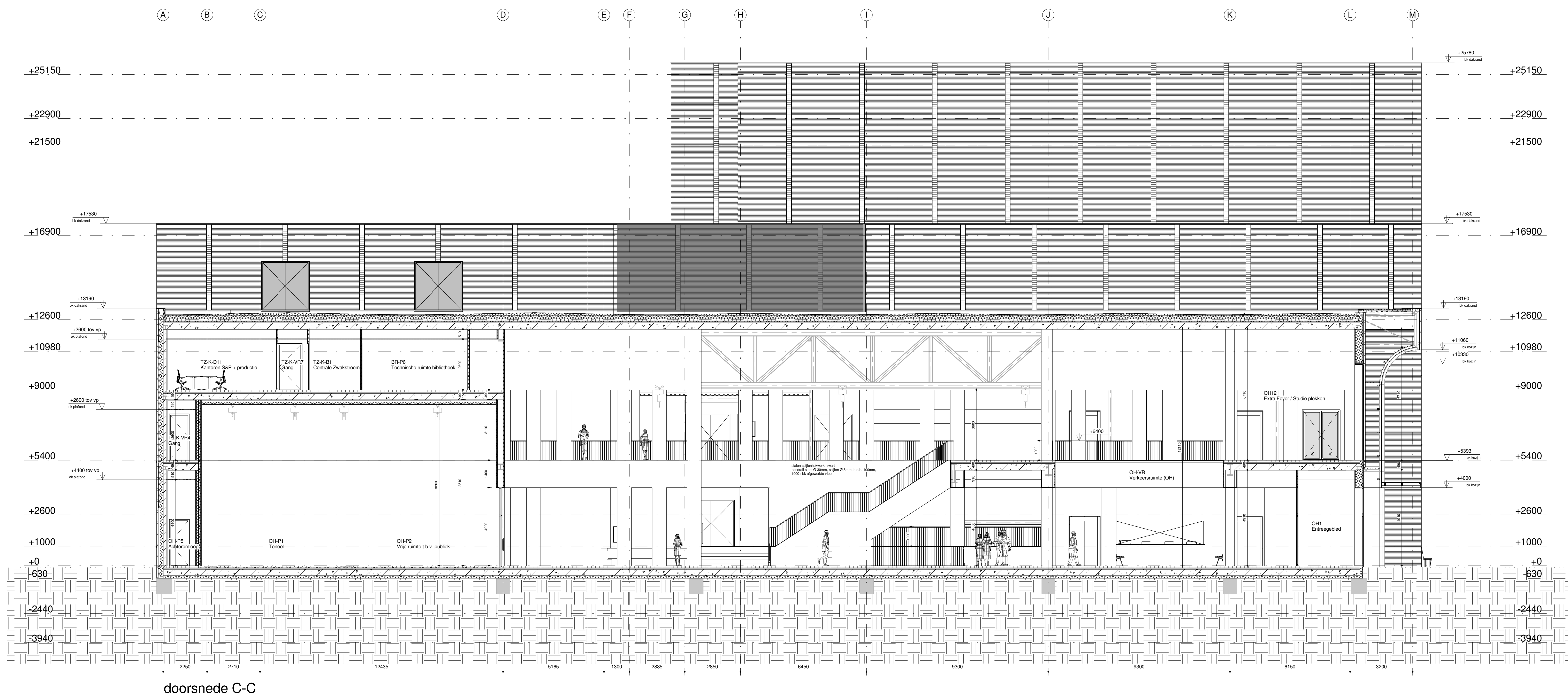
doorsnede C-C
