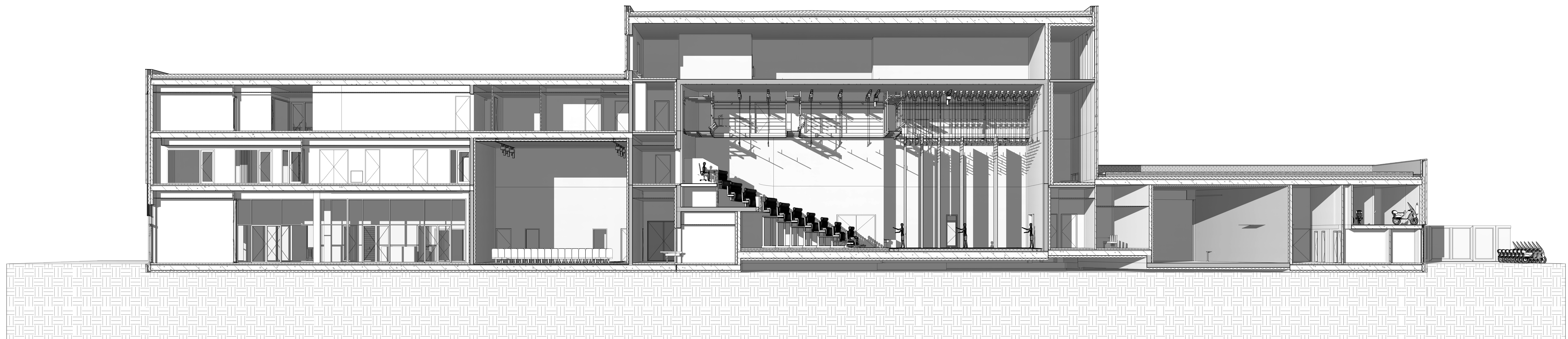
doorsnede A-A
