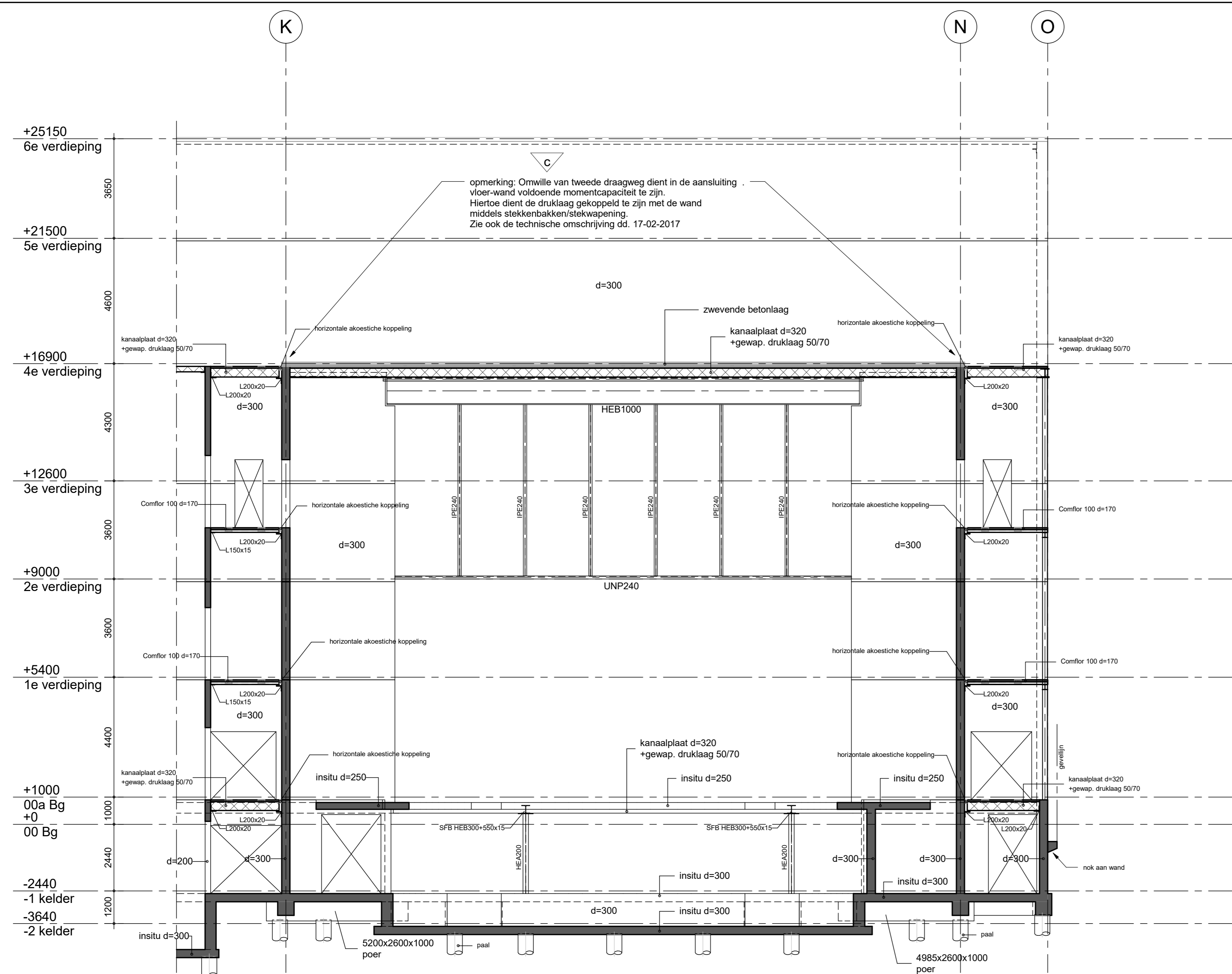
Doorsnede V3
