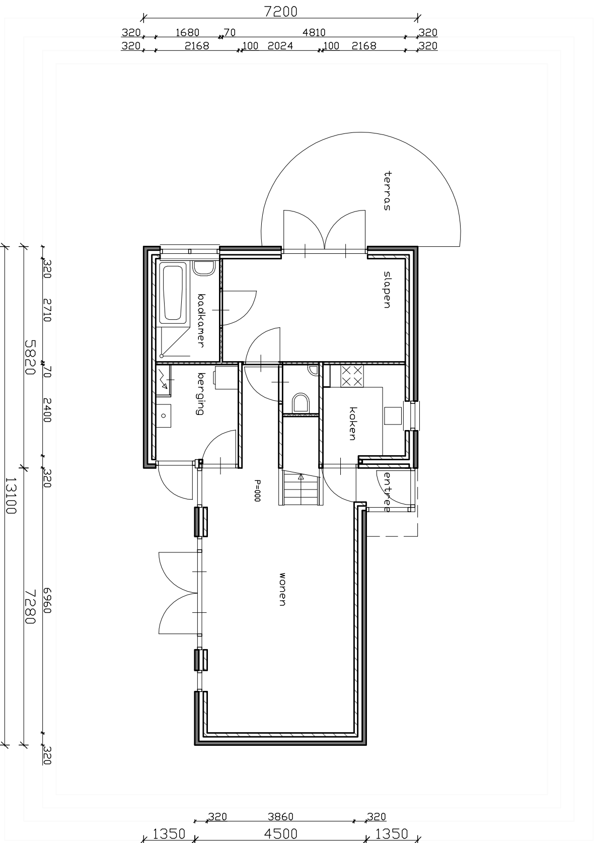
Begane grond
