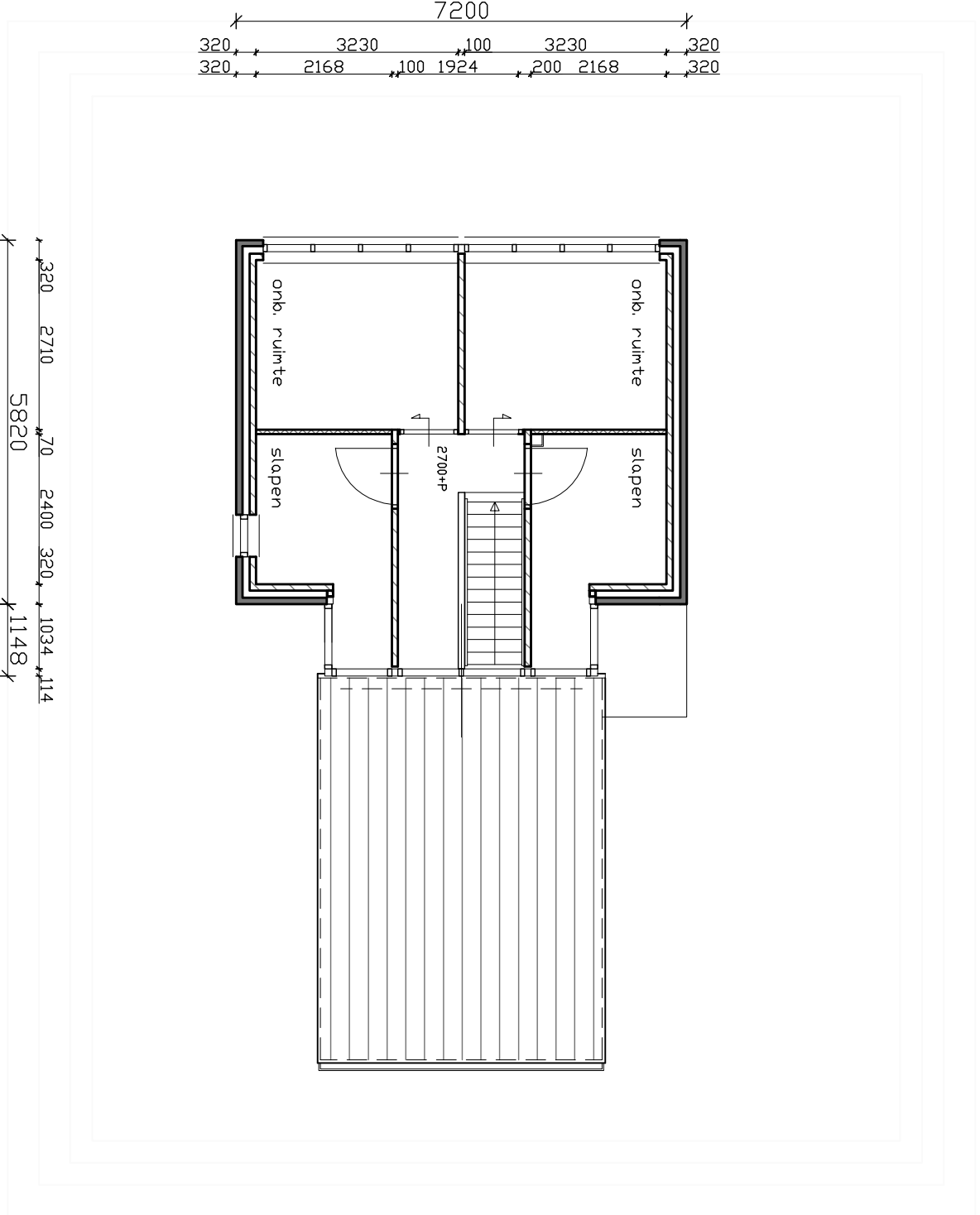
Verdieping
