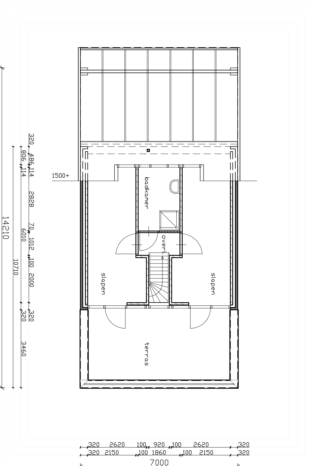
Verdieping
