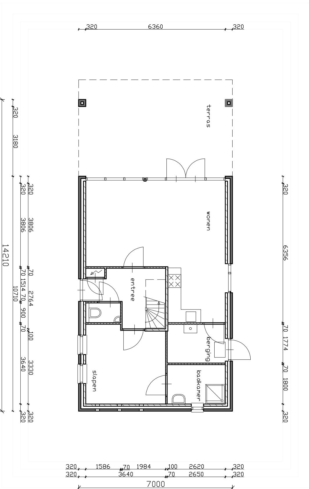
Begane grond
