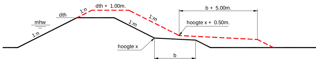
figuur 4: profiel van vrije ruimte wanneer afschuiven maatgevend is
