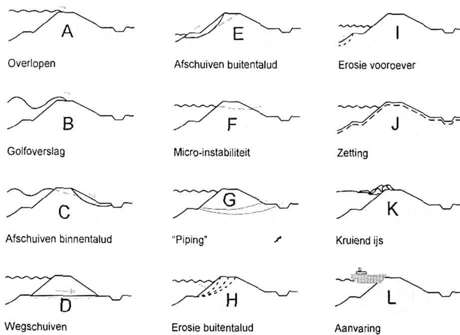
figuur 6: overzicht potentiële bezwijkmechanismen
