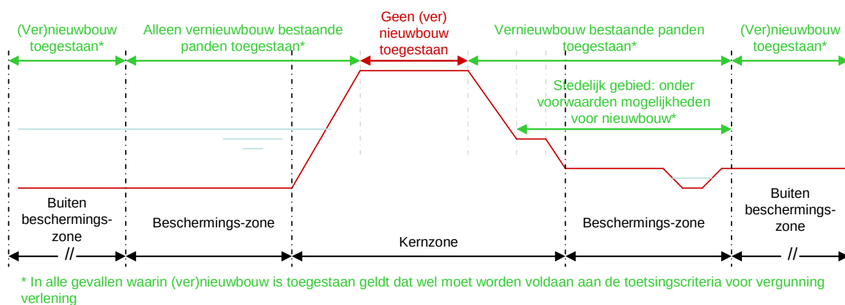
figuur 2: schematische weergave locatie-eisen bouwwerken
