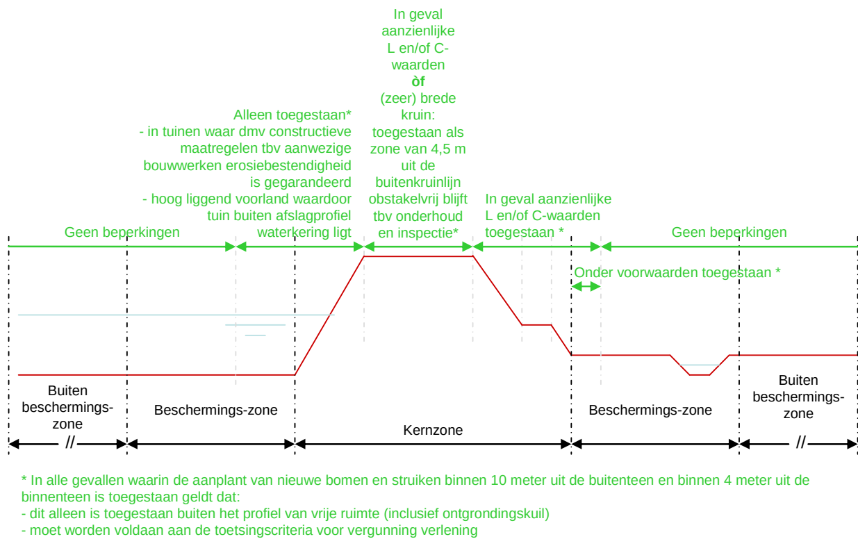
figuur 3: schematische weergave locatie-eisen aanplant nieuwe bomen en struiken
