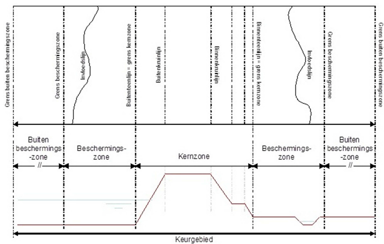
figuur 1: terminologie en zonering in het dwarsprofiel van een dijk
