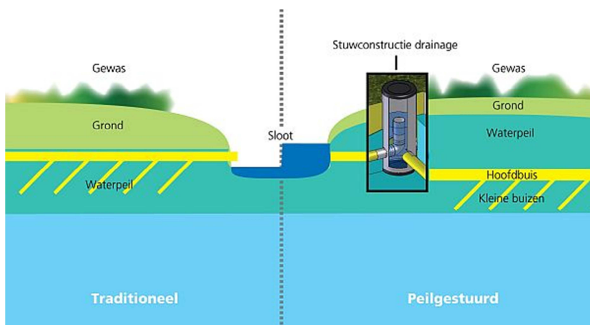
Conventionele drainage (links) versus peilgestuurde drainage (rechts)
