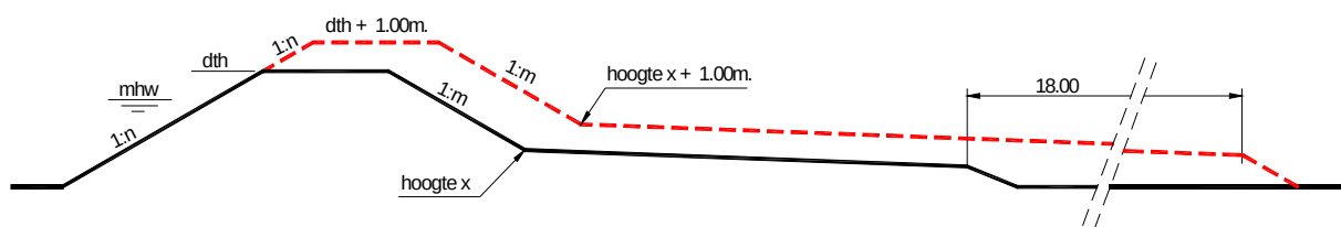
figuur 5: profiel van vrije ruimte wanneer piping/opbarsting maatgevend is
