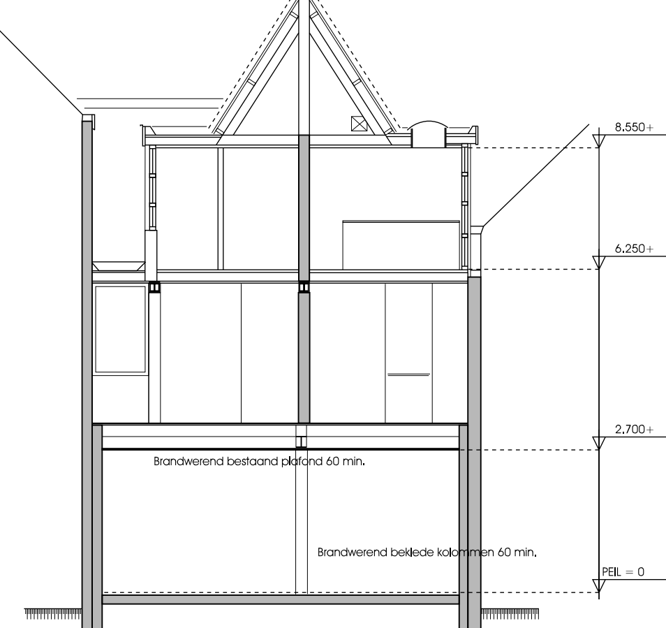
Bestaande doorsnede AA
