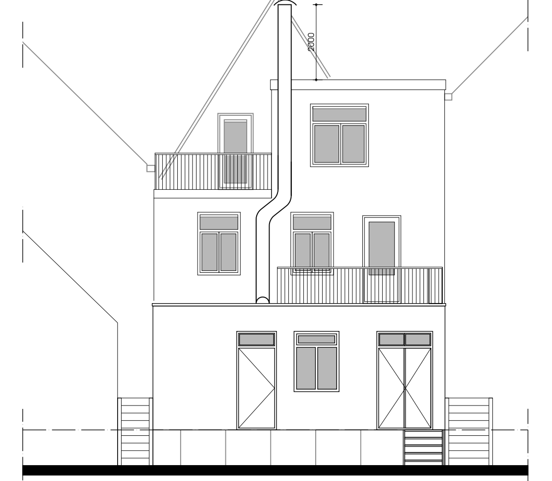
Achtergevel nieuw
