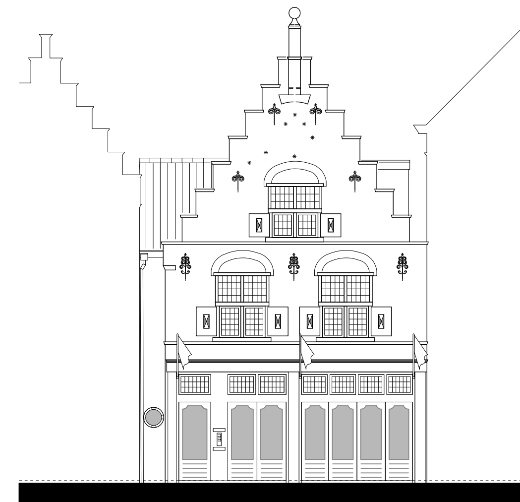
Gevel bestaand
