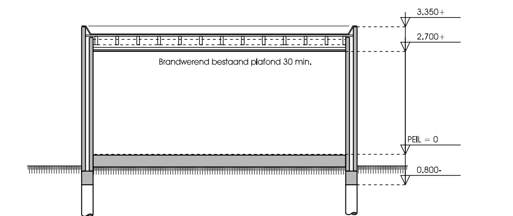
Bestaande doorsnede BB
