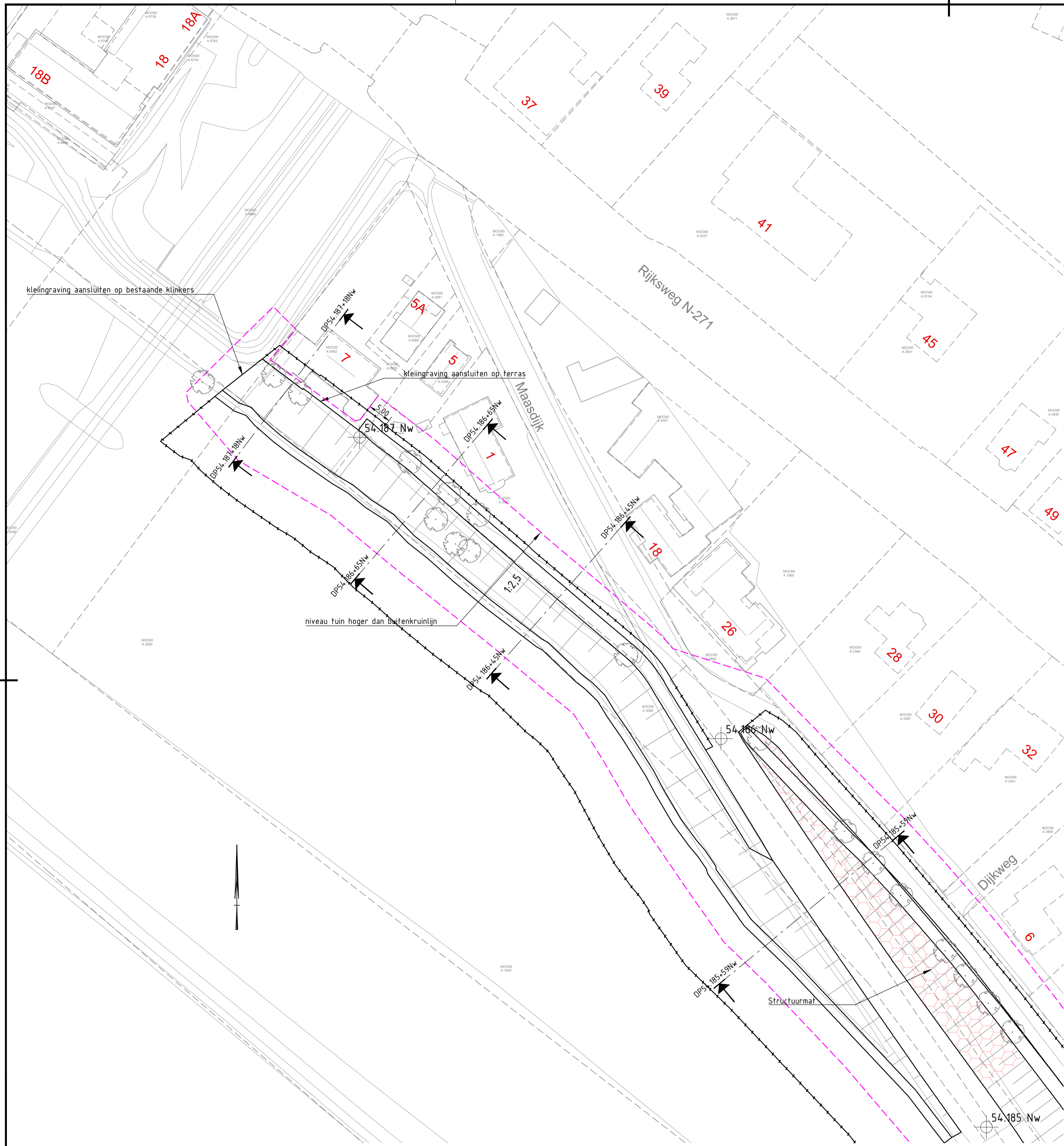
Situatie aansluiting grondlichaam spoorbrug Mook schaal 1:500
