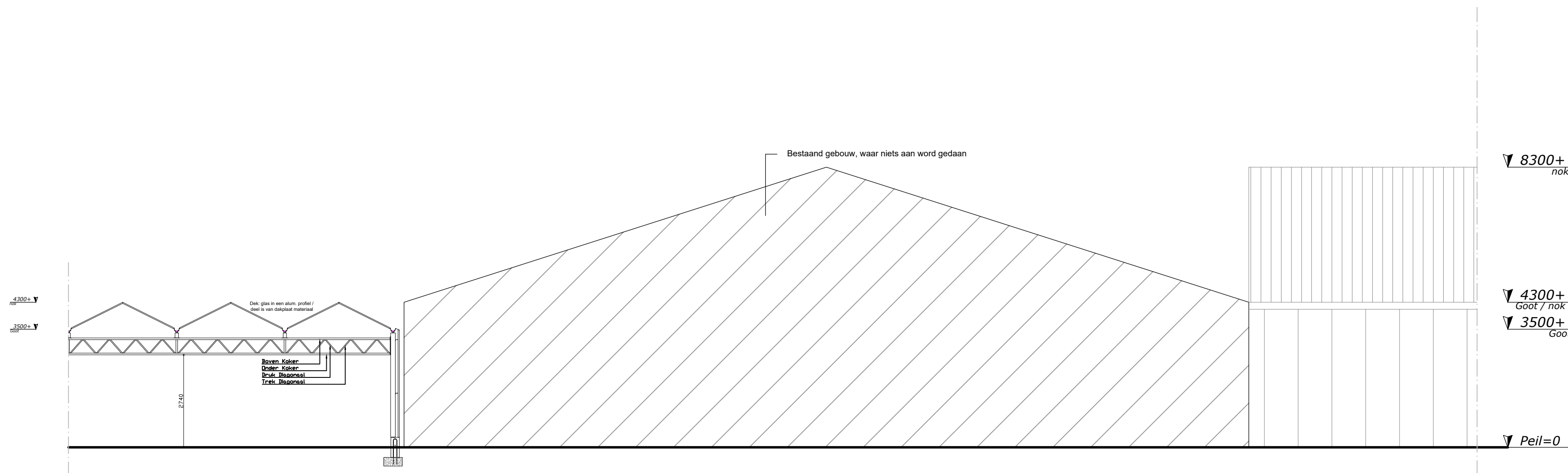
Doorsnede A-A Schaal: 1:100 Bestaande situatie
