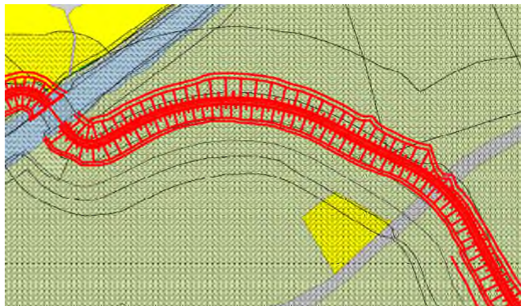
Figuur 2-5 Strijdigheid bestemmingsplan dijkvak 3 (legenda: Figuur 2-2)
