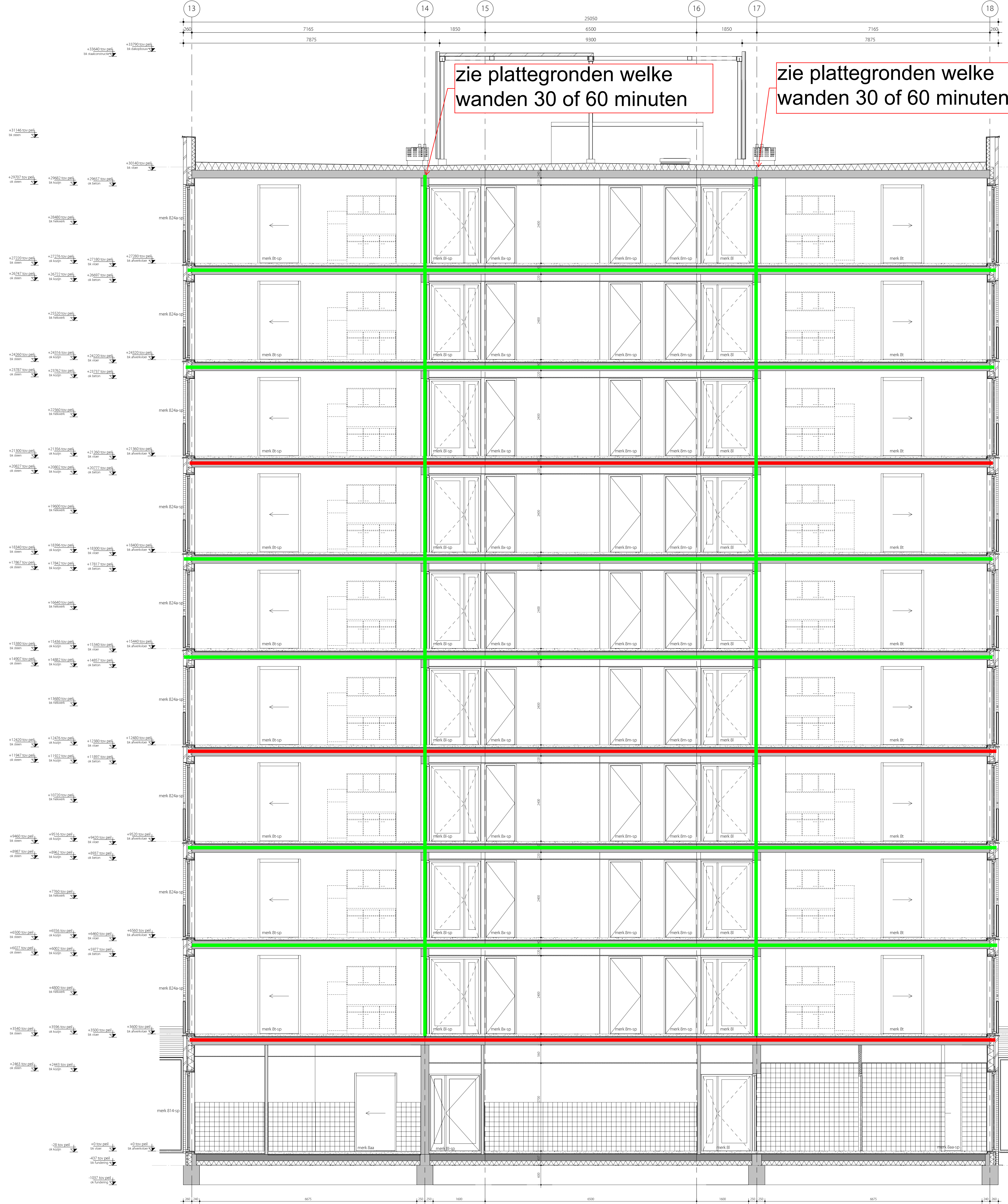
Doorsnede C
