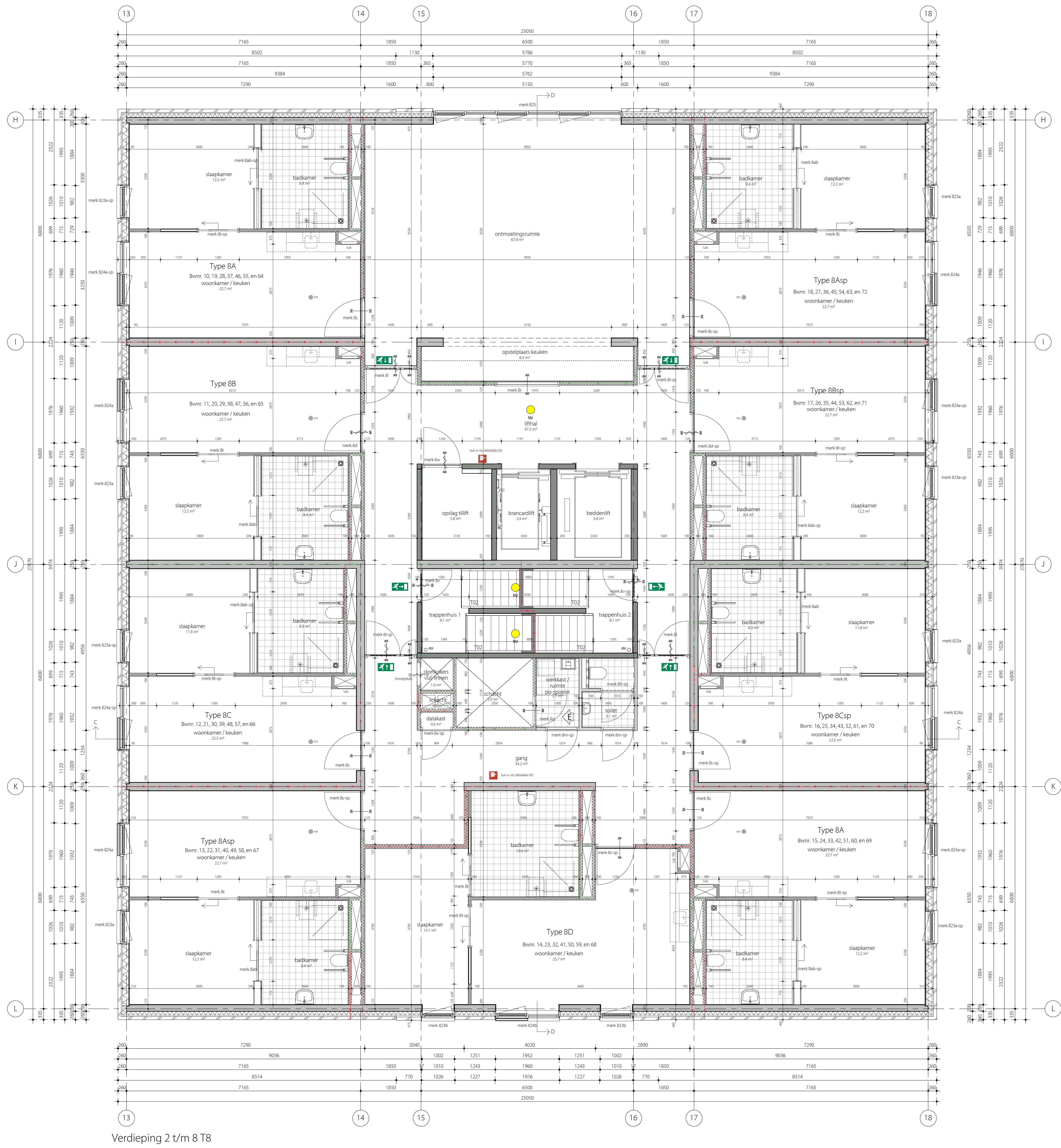
Verdieping 2 t/m 8 T8
