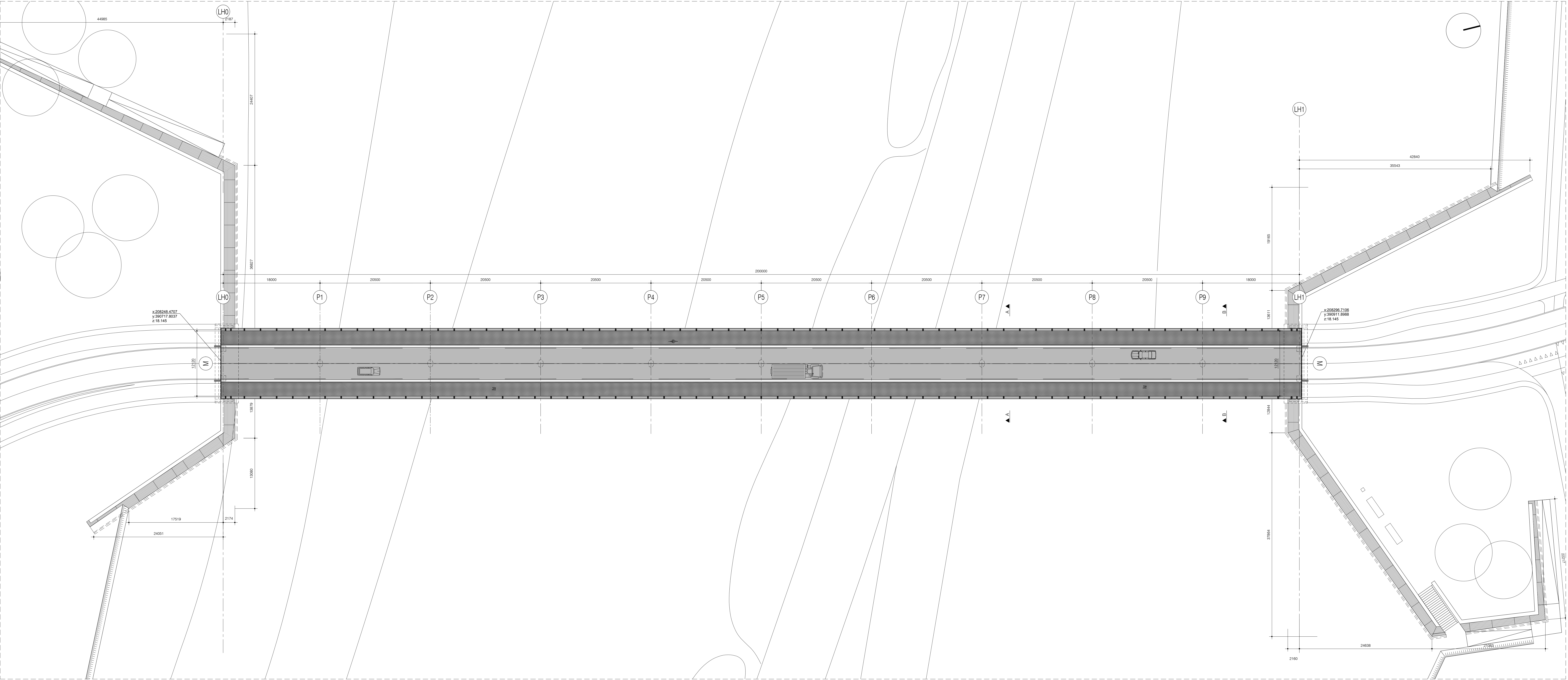
Planzicht Sch. 1:250
