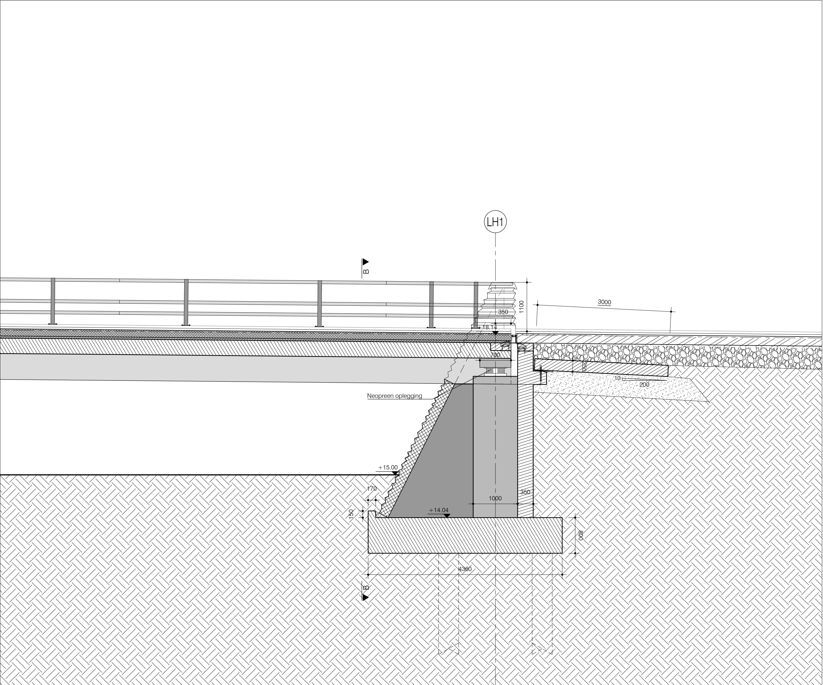
LH1: Snede A-A Schaal 1:50
