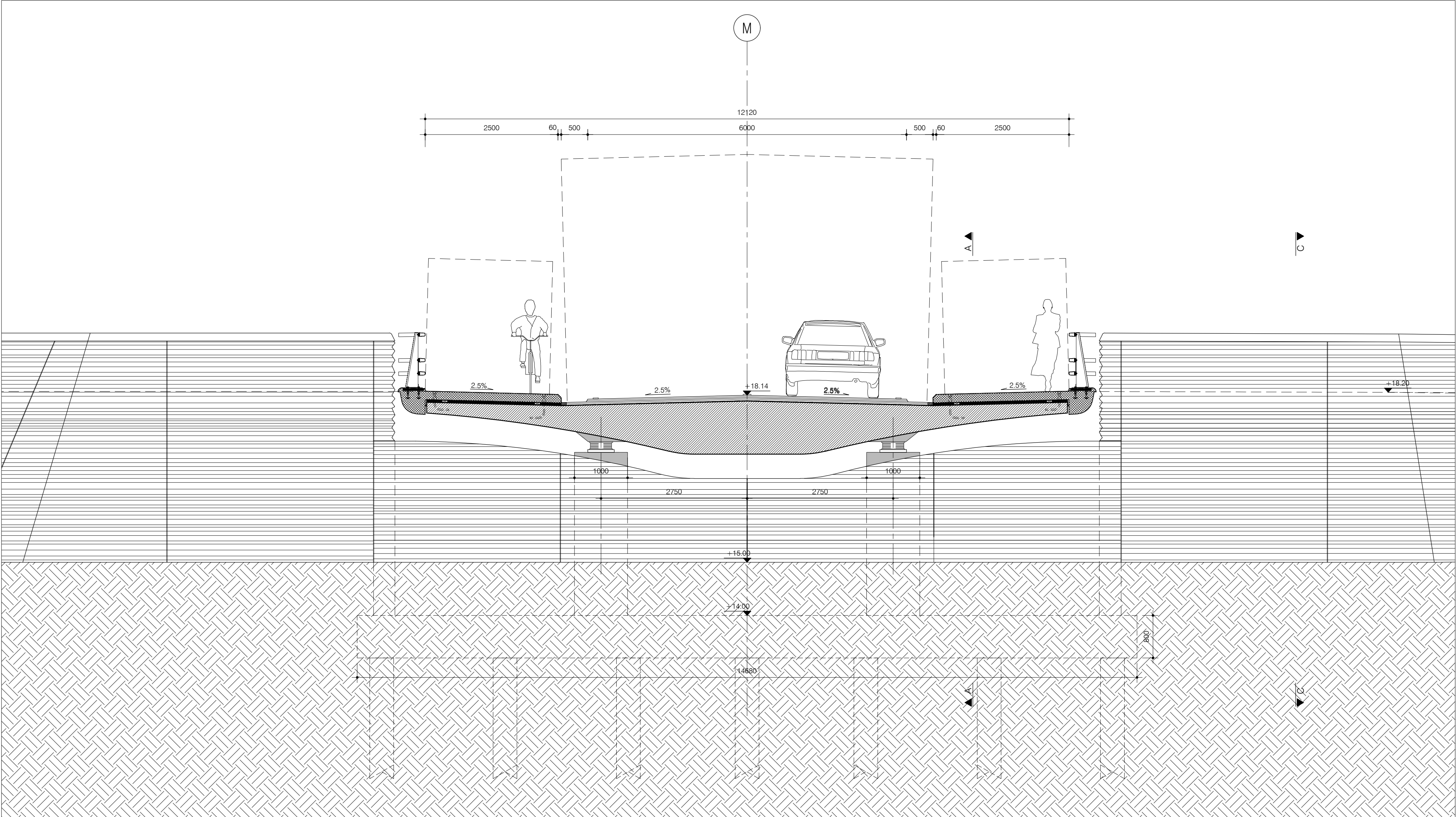
LH1: Snede B-B Schaal 1:50
