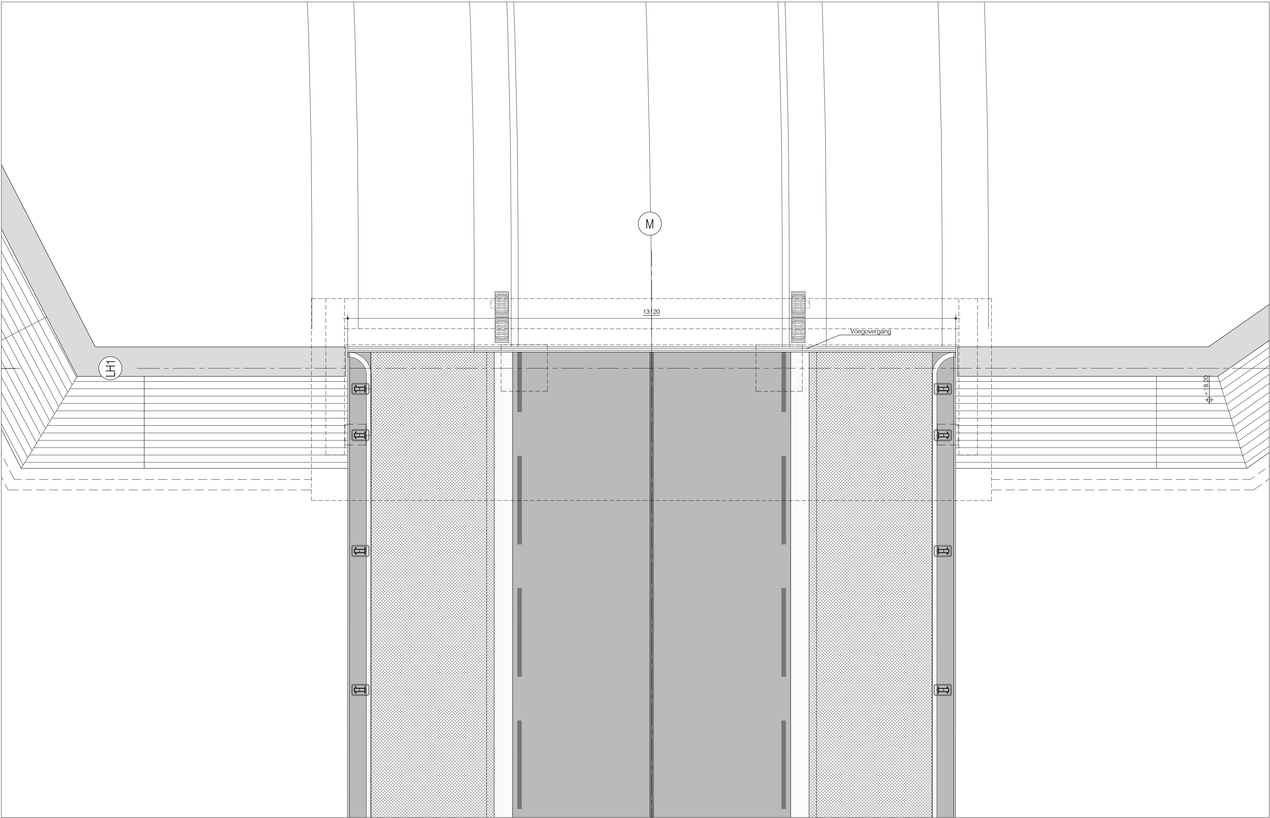
LH1: Planzicht Schaal 1:50
