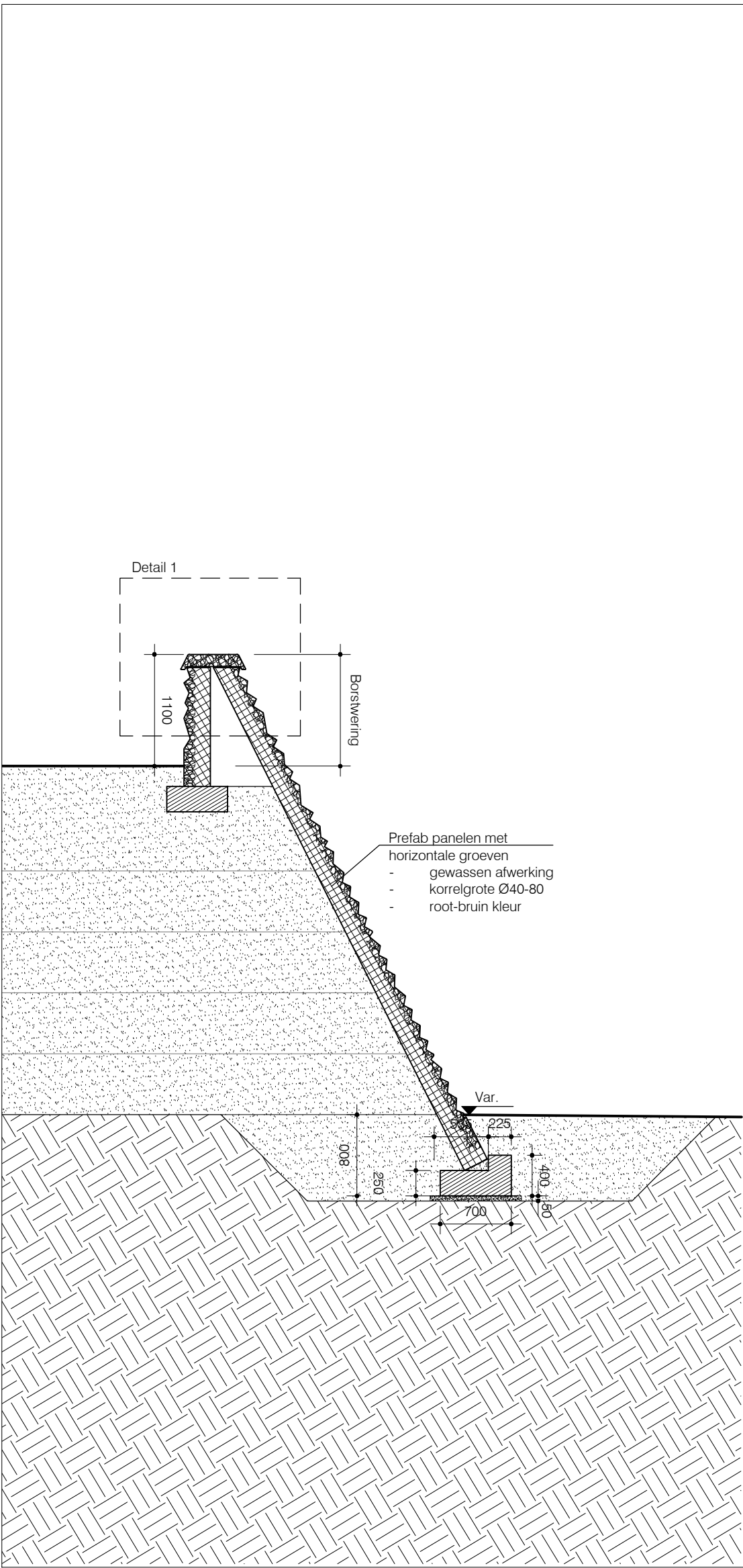
Typesnede C-C Schaal 1:50
