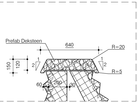
Detail 1 Schaal 1:20
